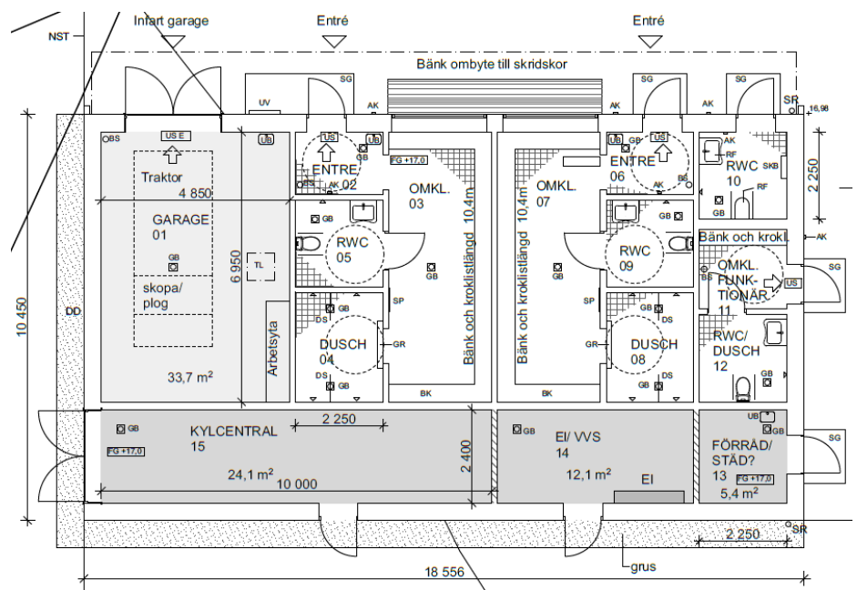
Planritning av planerad ny omklädningsbyggnad med garage och teknikutrymmen.
