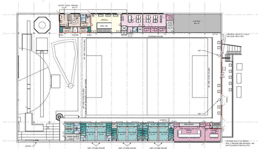
Planritning på övre plan. Rosa: teorirum och kansli, blå: omklädnings inomhusidrott, beige: personallokaler, gul: uppehållsytta, grå: teknik- och drifttytor. (Källa: Nyréns Arkitektkontor)
