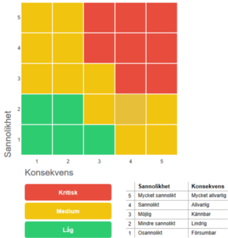
Bild 4: Riskmatrix
