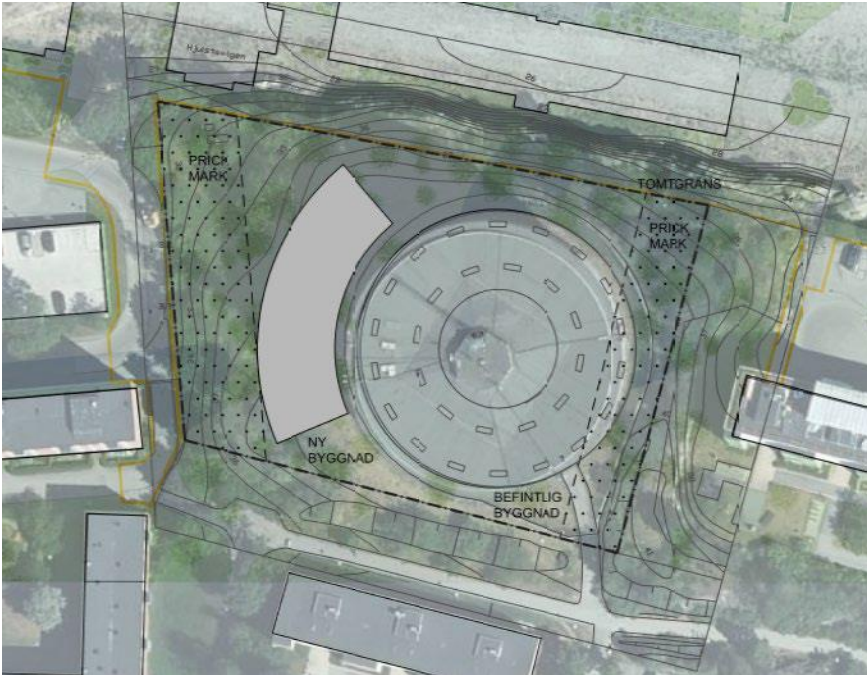
Figur 1. Ovan finns en skiss som visar det förslag som bedöms vara det bästa för att komplettera med ny reservoarvolym.
