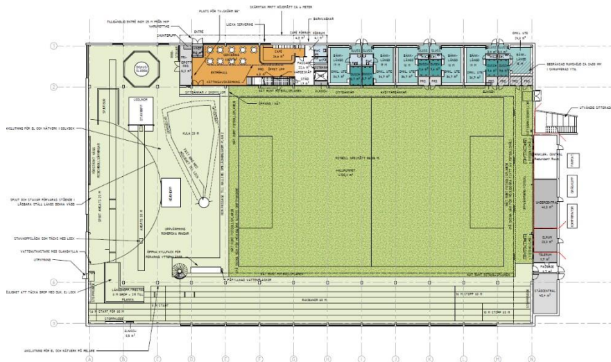
Planritning på entréplan. Ljusgrön: fridrottsytor, mörkgrön: bollplan, orange: entréhall och kafé, blå: omklädning uteidrott, grå: teknik- och driftytor. (Källa: Nyréns Arkitektkontor).
