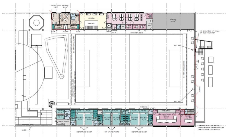
Planritning på övre plan. Rosa: teorirum och kansli, blå: omklädnings inomhusidrott, beige: personallokaler, gul: uppehållsyta, grå: teknik- och driftytor. (Källa: Nyréns Arkitektkontor)
