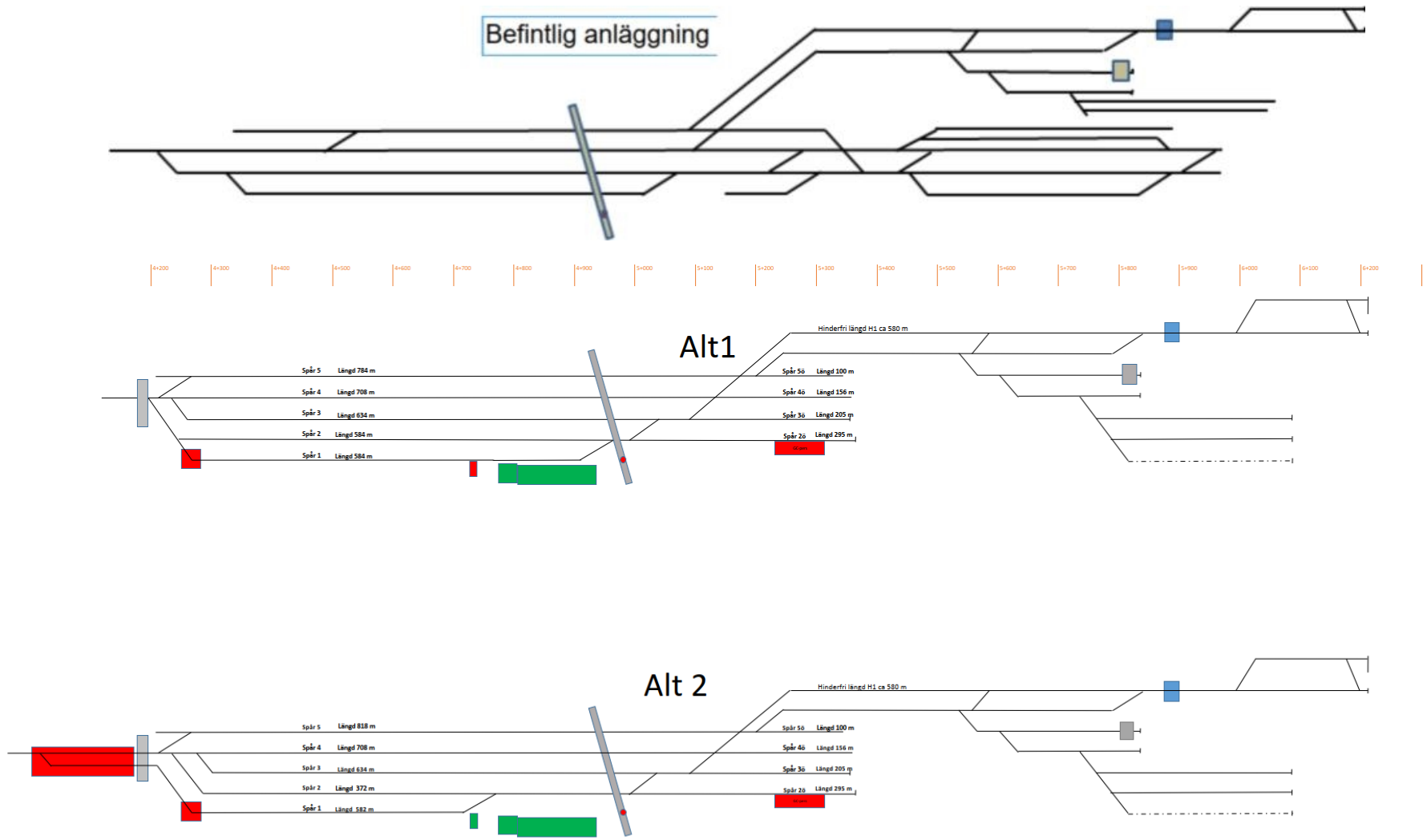
Bilaga1: Schematisk skiss utredningens spårutformningar dat.2020-01-17
