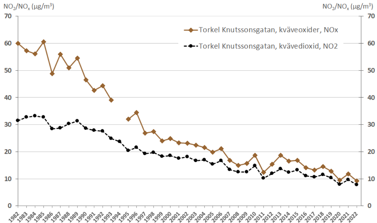
Figur 2. Trender för årsmedelvärden av kväveoxider, NO x , och kvävedioxid, NO 2 , för perioden 1982–2022 i Stockholms urbana bakgrundsluft som mäts i taknivå vid Torkel Knutssonsgatan.
