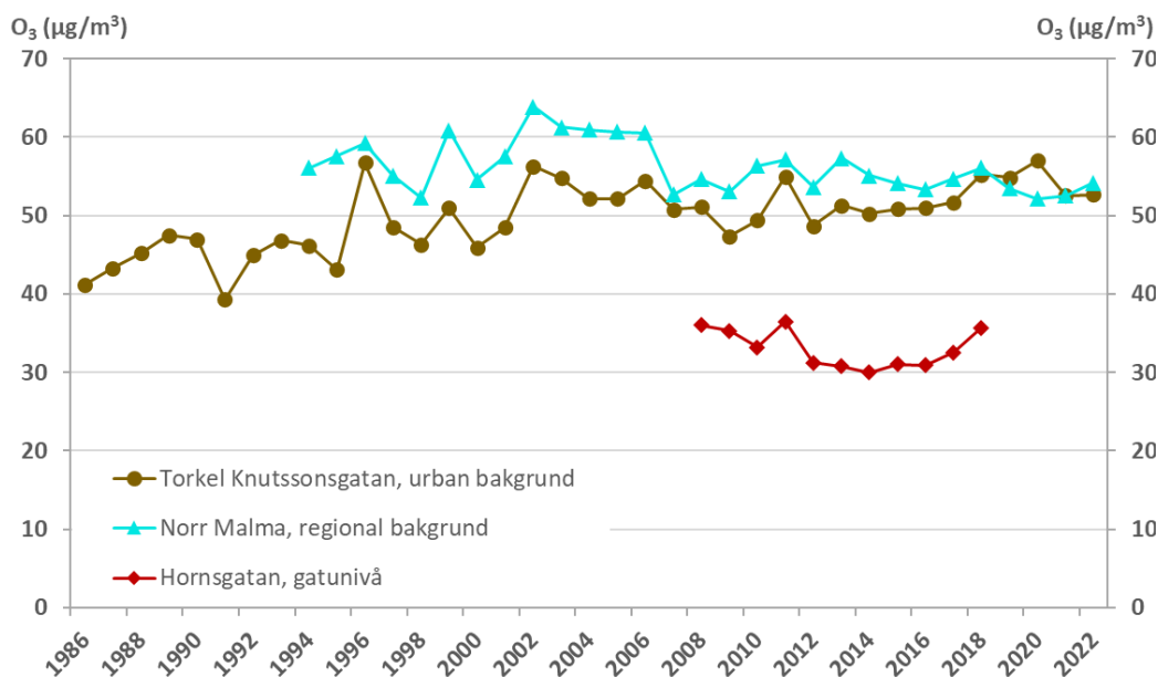
Figur 13. Trender för årsmedelvärden av ozon för perioden 1986–2022.
