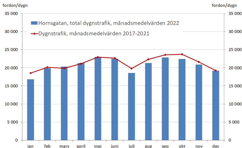
Figur 19. Månadsmedelvärden av trafikflöden på Hornsgatan år 2022. Jämförelse med medelvärdet för femårsperioden 2017 t.o.m. 2021.
