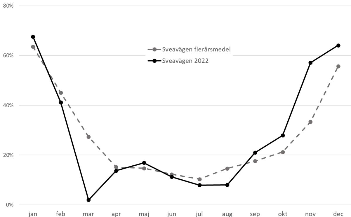
Figur 17. Uppmätta månadsmedelvärden för antal timmar med fuktig vägbana på Sveavägen år 2022 samt jämförelse med flerårsmedelvärdet 2014–2021.
