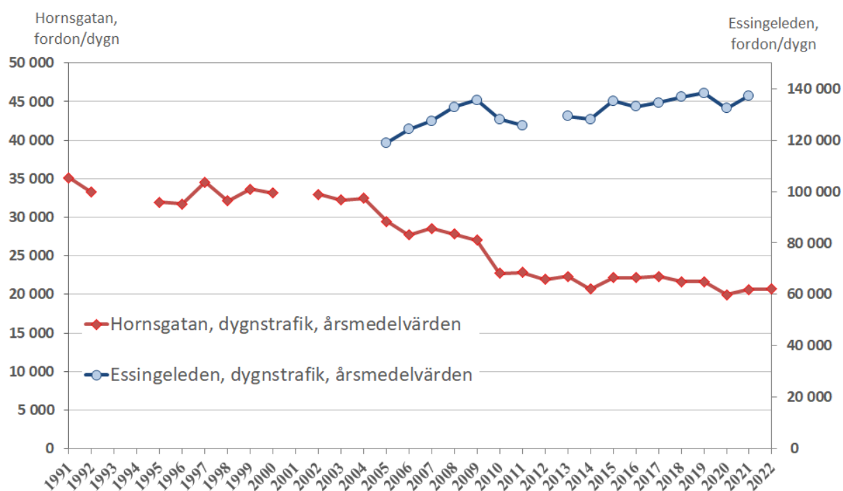
Figur 21. Trender för trafikmängder (fordon/dygn) på Hornsgatan 1991–2022 (vänster axel) och E4/E20 Essingeleden 2005–2021 (höger axel). Årsvärde 2022 saknas för E4/E20 Essingeleden p.g.a. att data för november och december inte är klara.
