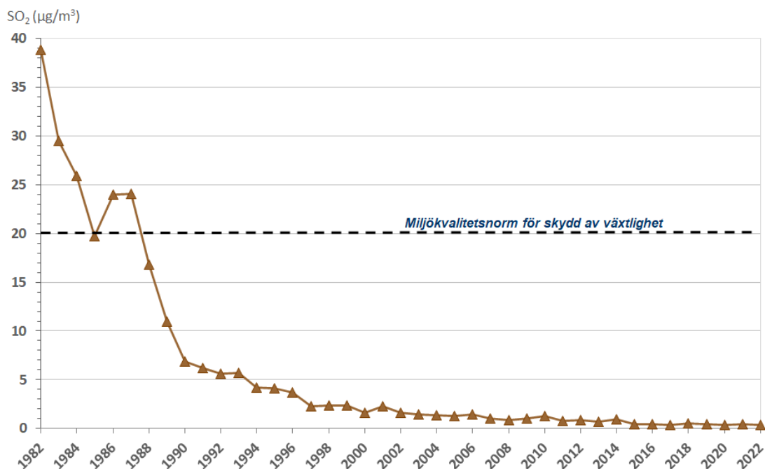
Figur 12. Trend för svaveldioxid, SO 2 , årsmedelvärden vid mätstationen i urban bakgrund vid Torkel Knutssonsgatan under perioden 1982–2022. Jämförelse med miljö kvalitetsnorm till skydd av växtlighet.
