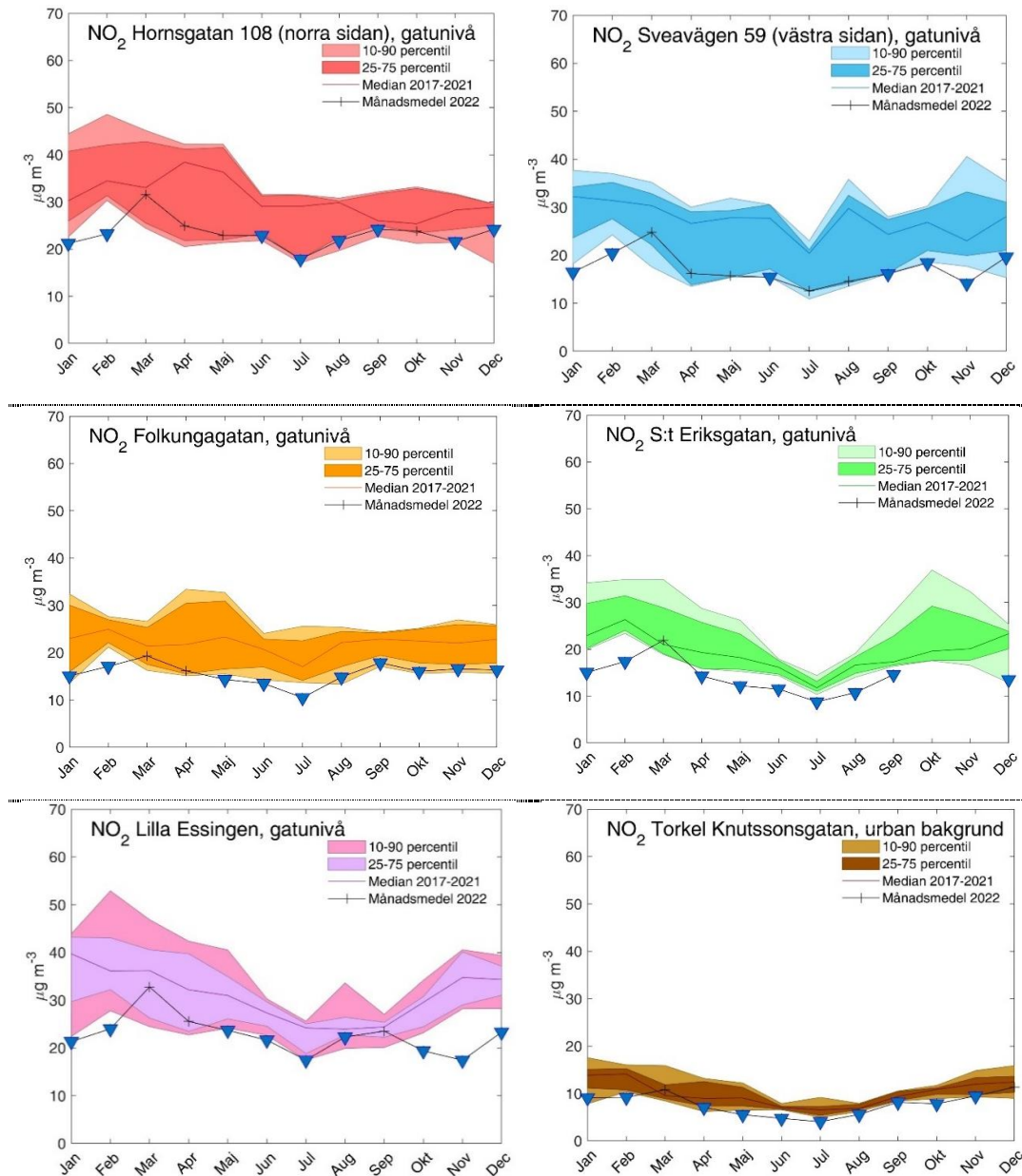
Figur 1. Kvävedioxid, NO 2 , månadsmedelvärden år 2022 i jämförelse med medelvärden 2017 t.o.m. 2021 (färgade fält). Blå triangel indikerar tydligt lägre månadsmedelvärde år 2022.
