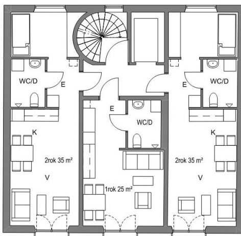
Exempel på normalplan i tillkommande byggnad. Bild: Lugnet Arkitektur.
