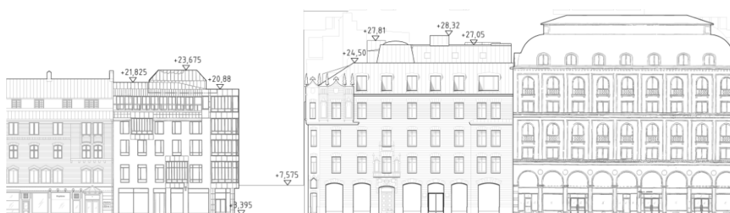
Fasadelevation mot Biblioteksgatan (nedre bild) med rekonstruerad sockelvåning, samrådsförslag.
