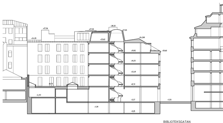
Sektion som visar kontorsdelen mot Biblioteksgatan samt underbyggd gård.
