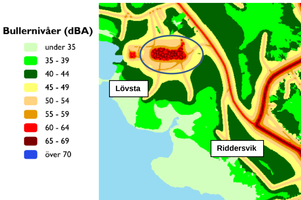
Figur 3. Stockholm stads bullerkarta där samtliga bullerkällor är medräknade (väg, spår, flyg och industri) ekvivalent, dygn. Ungefärlig placering av återvinningscentralen inom blå ellips. Källa: Stockholm stad, 2018
