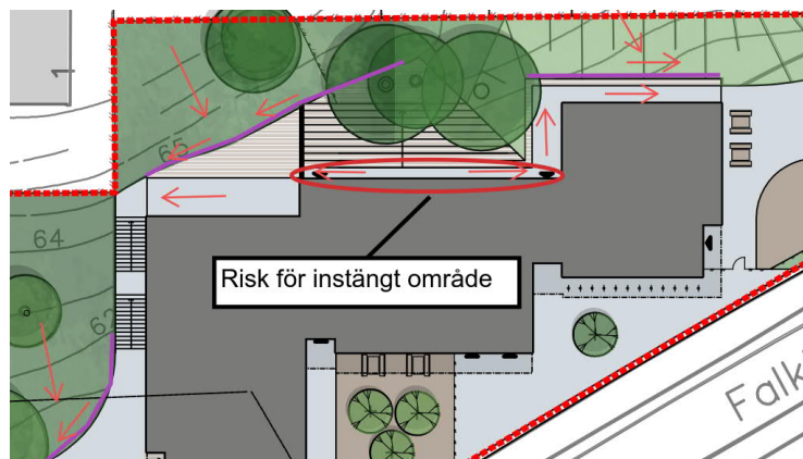
Figur 5. Mellan byggnaden och naturmarken krävs extra omsorg vid höjsättningen för att inte skapa instängda områden där dagvattnet kan bli stående och svämma över mot byggnaden.
