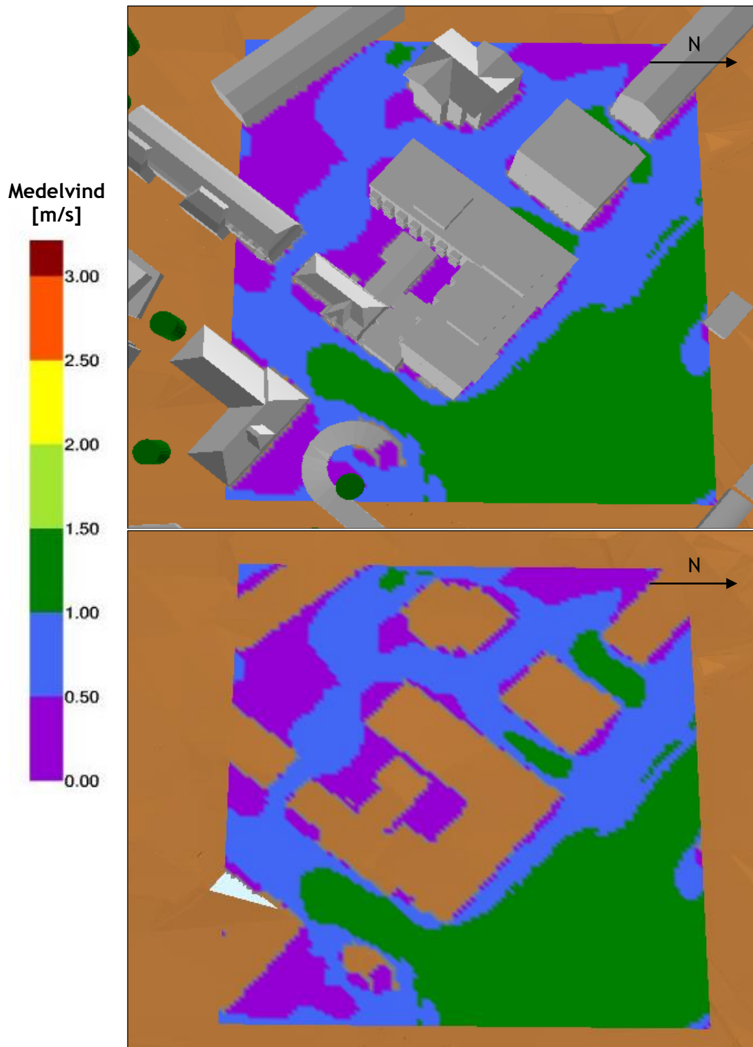
Figur 8: Medelvindförhållande under året, 2 m över marken. Överst visas förhållande med samtliga byggnader. Nederst utan byggnader för att tydliggöra vindförhållandena runt byggnaderna.
