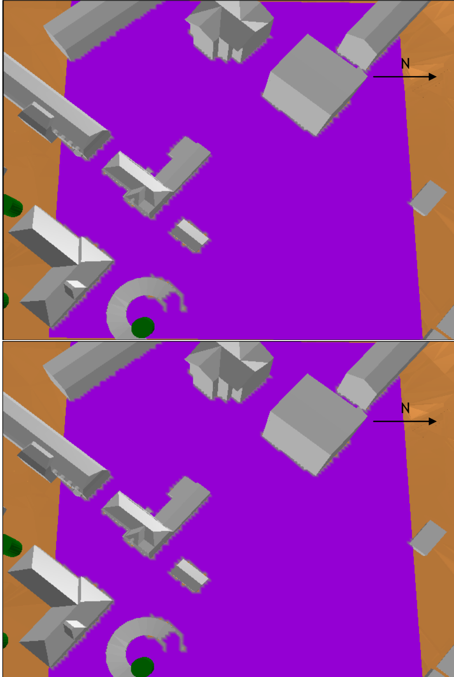
Figur 17: Områden som uppfyller kravet medelvind över 5,5 m/s högst 1 % av tiden, före bygget av Spånga Studios. Översikt för sommarhalvåret (överst) och vinterhalvåret (nederst). Figuren är analog till Figur 11 (med Spånga Studios).
