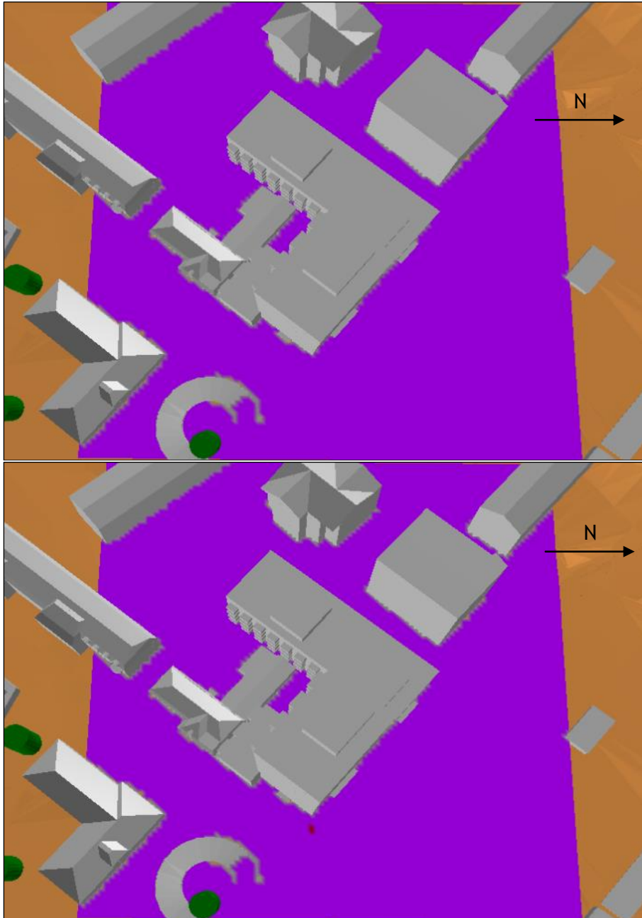
Figur 12: Områden som uppfyller kravet medelvind över 5,5 m/s högst 1 % av tiden. Översikt för områdena runt Spånga Studios, för sommarhalvåret (överst) och vinterhalvåret (nederst).
