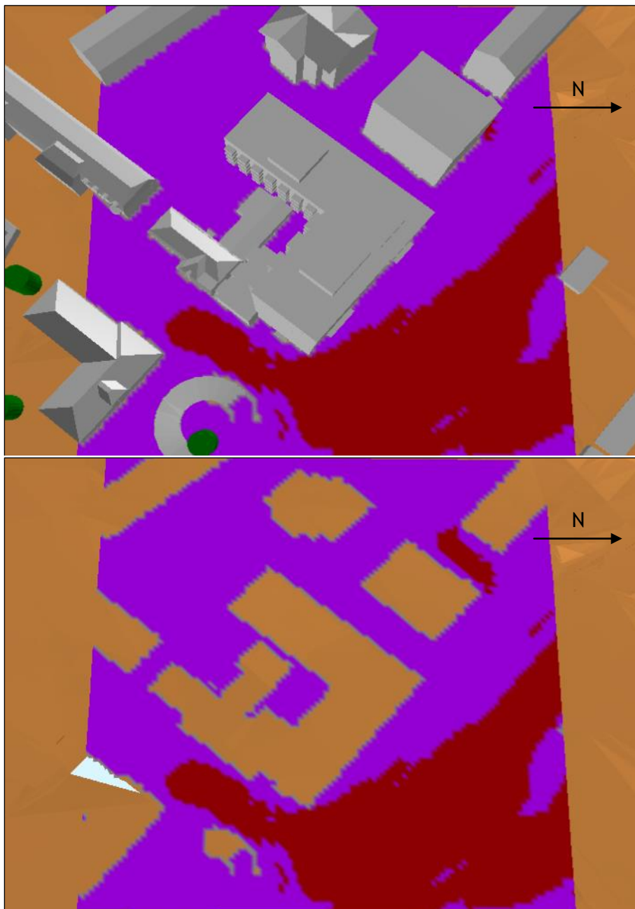
Figur 11: Områden som uppfyller kravet medelvind över 3,5 m/s högst 4 % av tiden. Översikt för områdena runt Spånga Studios, för vinterhalvåret. Nederst visas vinden utan samtliga byggnader för att tydliggöra vindförhållanden runt om byggnaden.
