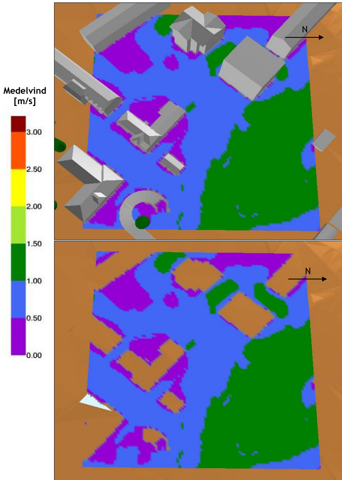
Figur 14: Pre Spånga Studios. Medelvindförhållande under året, 2 m över marken. Överst visas förhållande med samtliga byggnader. Nederst utan byggnader för att tydliggöra vindförhållandena runt byggnaderna. Figuren är analog till Figur 8 (med Spånga Studios).
