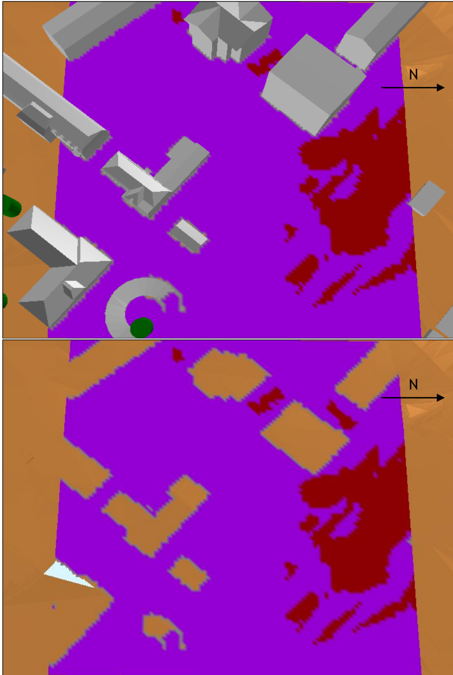
Figur 16: Områden som uppfyller kravet medelvind över 3,5 m/s högst 4 % av tiden, före bygget av Spånga Studios. Översikt för vinterhalvåret. Nederst visas vinden utan samtliga byggnader för att tydliggöra vindförhållanden runt om byggnaden. Figuren är analog till Figur 10 (med Spånga Studios).
