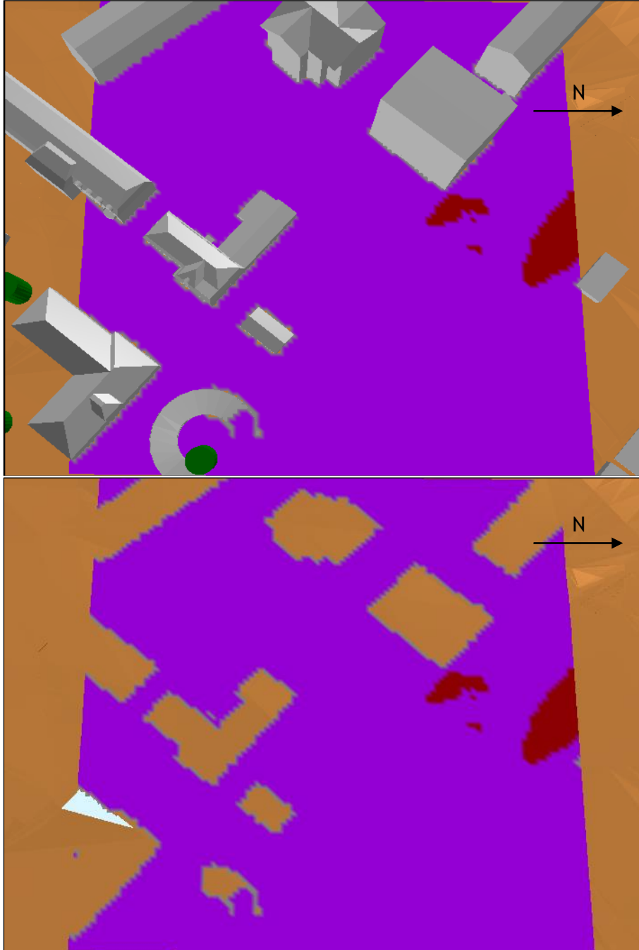
Figur 15: Områden som uppfyller kravet medelvind över 3,5 m/s högst 4 % av tiden, före bygget av Spånga Studios. Översikt för sommarhalvåret. Nederst visas vinden utan samtliga byggnader för att tydliggöra vindförhållanden runt om byggnaden. Figuren är analog till Figur 9 (med Spånga Studios).
