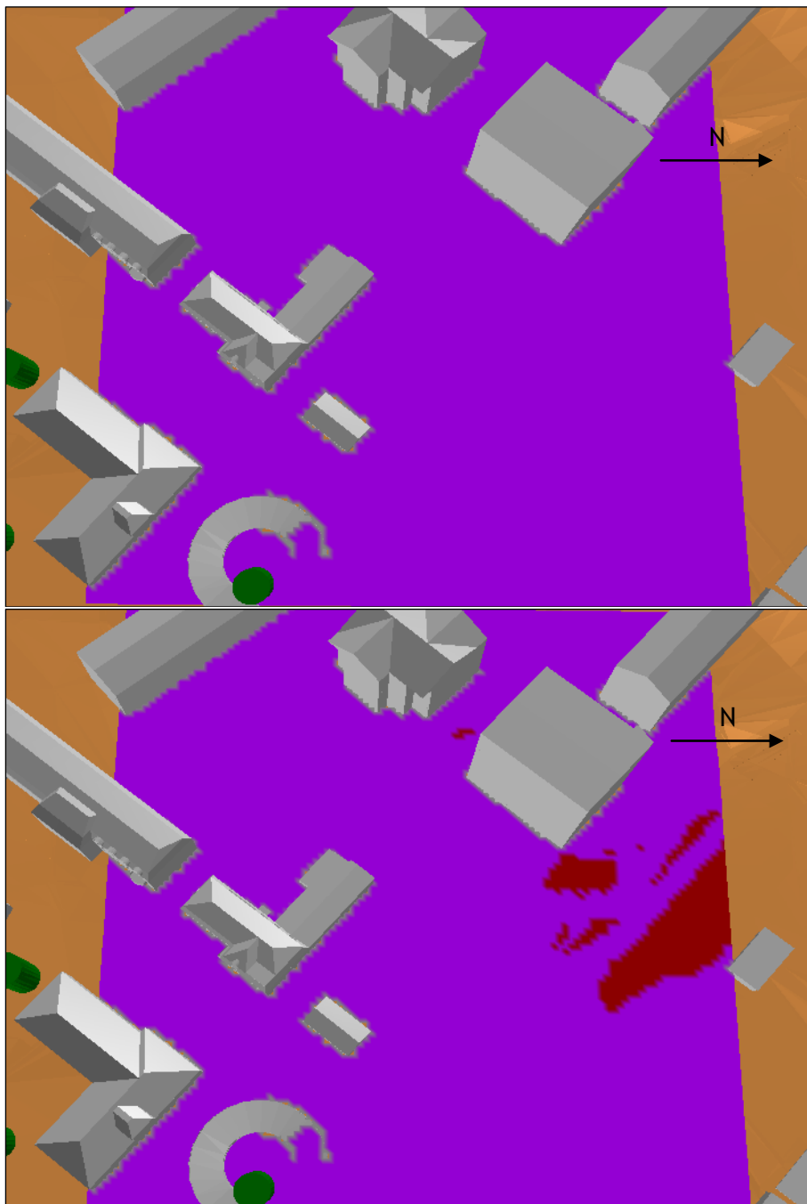
Figur 18 Områden som uppfyller kravet medelvind över 3,5 m/s högst 6 % av tiden, före bygget av Spånga Studios. Översikt för sommarhalvåret (överst) och vinterhalvåret (nederst). Figuren är analog till Figur 12 (med Spånga Studios).
