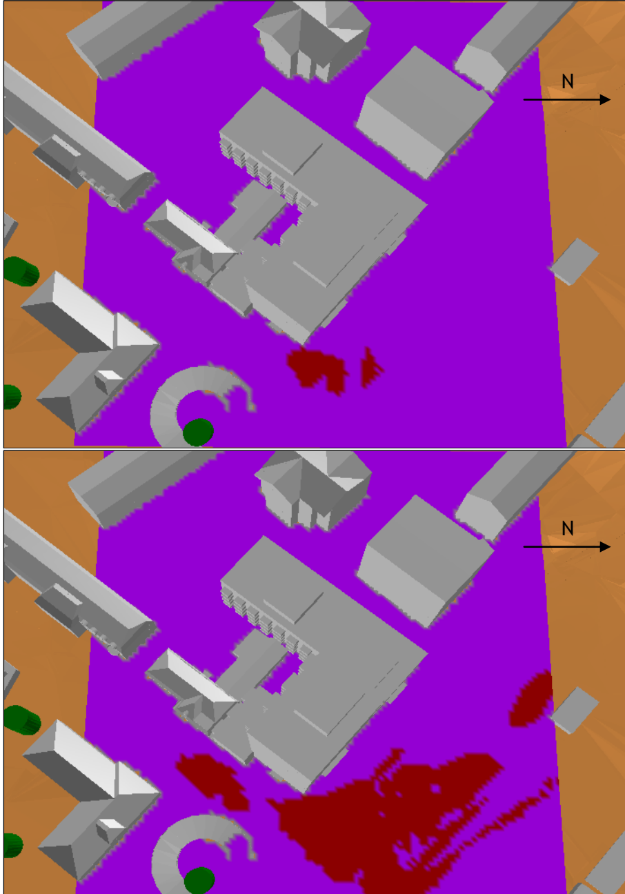
Figur 13: Områden som uppfyller kravet medelvind över 3,5 m/s högst 6 % av tiden. Översikt för områdena runt Spånga Studios, för sommarhalvåret (överst) och vinterhalvåret (nederst).
