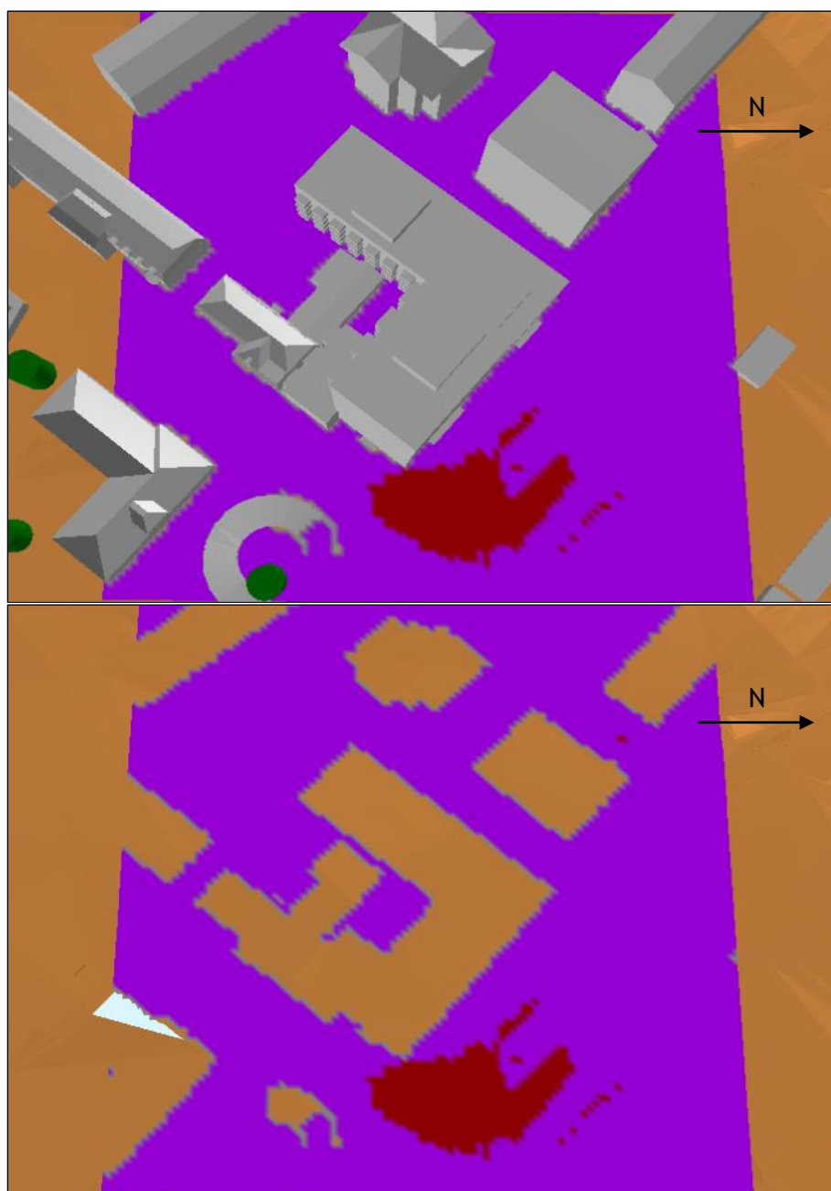
Figur 10: Områden som uppfyller kravet medelvind över 3,5 m/s högst 4 % av tiden. Översikt för områden runt Spånga Studios, för sommarhalvåret. Nederst visas vinden utan samtliga byggnader för att tydliggöra vindförhållanden runt om byggnaden.
