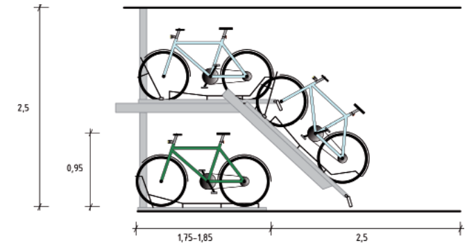
Plats för tvåvåningsställ. Minimihöjden i cykelparkeringen bör vara 2,5 meter, gången mellan cykelställ minst 2,5 meter. Källa: Cykelparkering i staden, Trafikkontoret Stockholms stad.
