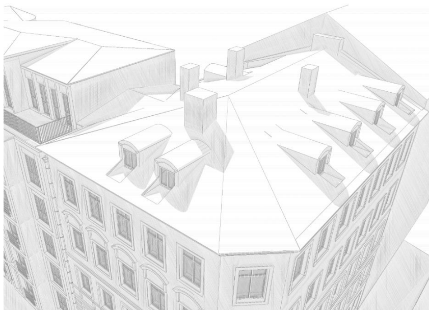
Illustration som visar de sju nya takkupornas placering. Kuporna ska ha välvd takprofil och vara väl indragna. Halvorsen Coast
