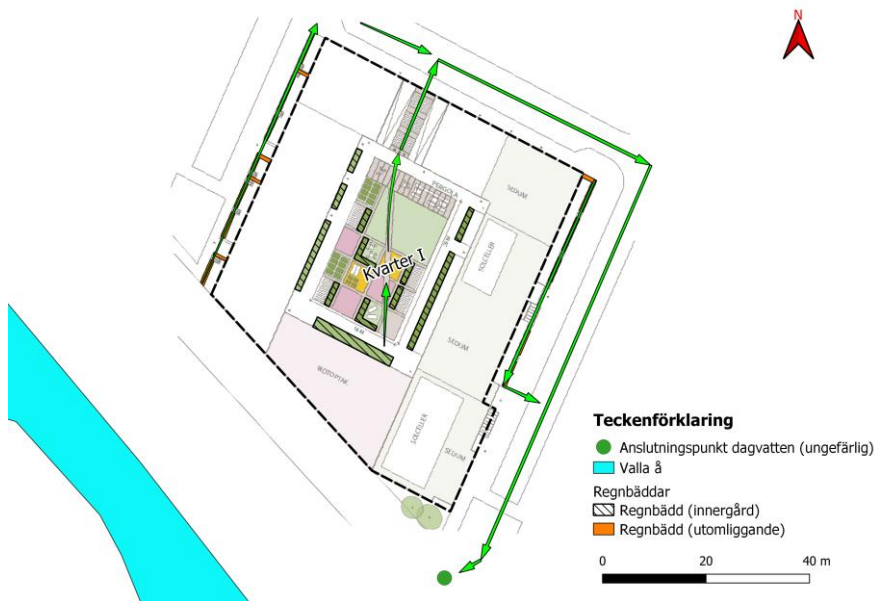
Figur 13-2. Exempel på hur dagvatten från regnbäddar leds via ledningsnät för dagvatten från Kvarter I mot befintlig anslutningspunkt för dagvattensystemet.
