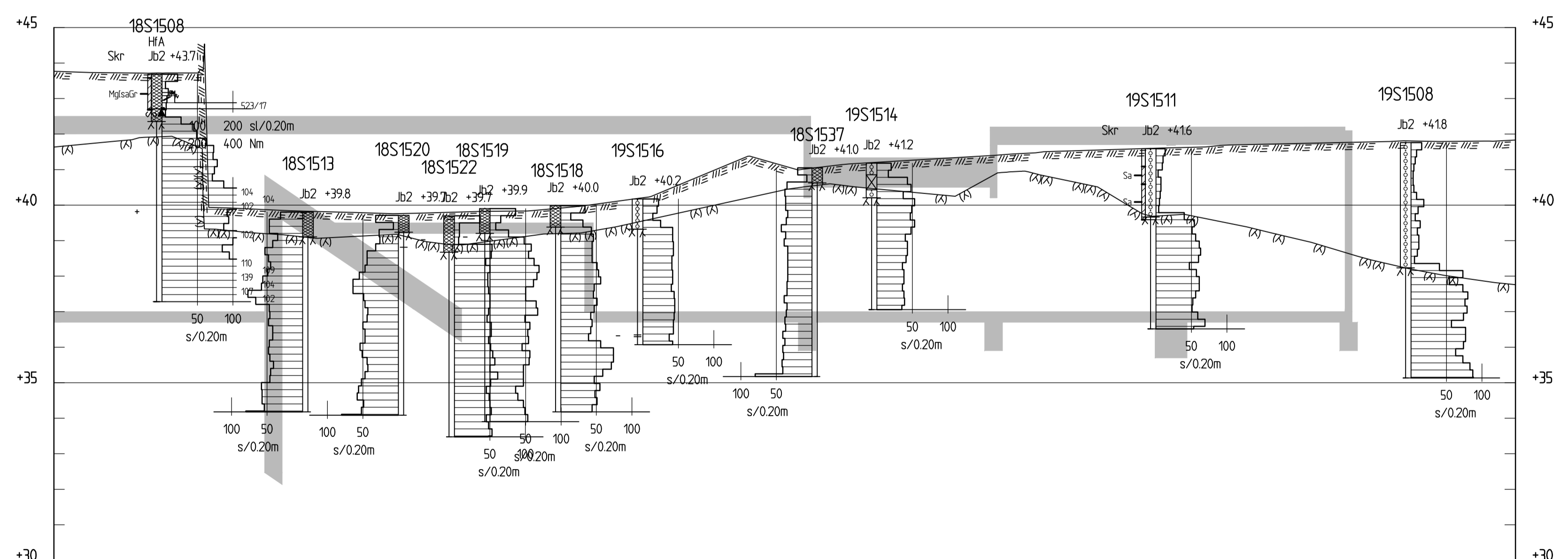
SEKTION B-B H 1: 100 L 1: 200
