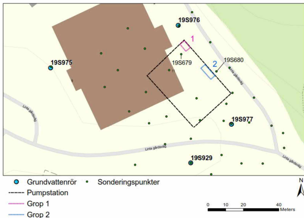
Figur 2 Pumpstationens läge och befintliga grundvattenrör. Läge för hopkoppling med ledningar markerade som Grop 1 och Grop 2.
