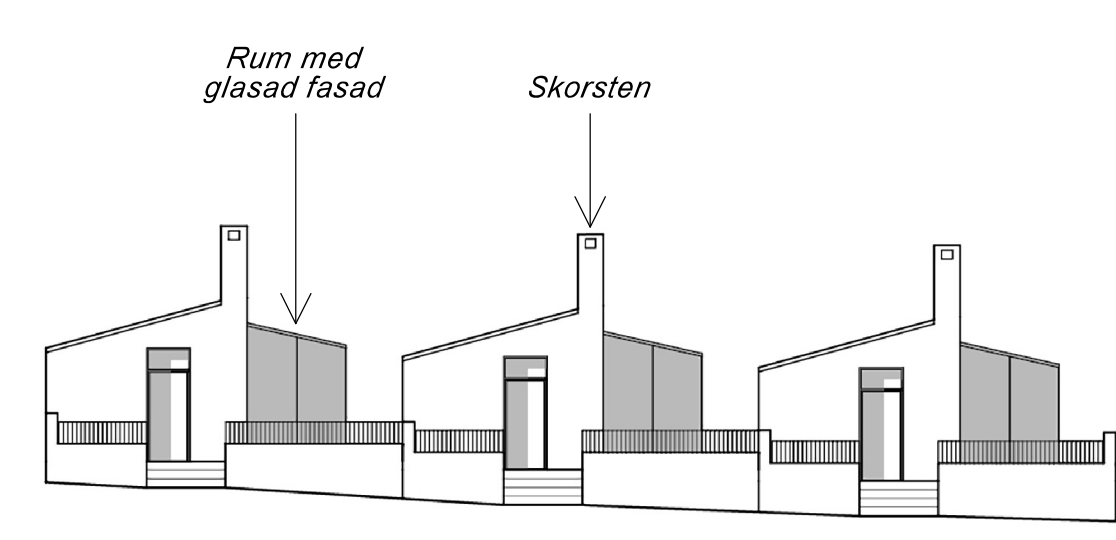
Illustration: Princip för volymer och fönstersättning mot norr.
