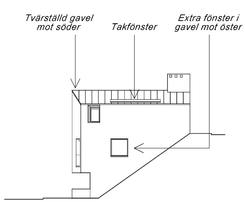
Illustration: Princip för volymer och fönstersättning på gavlar mot öster.
