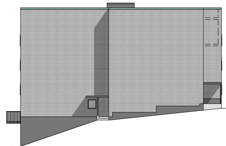
Befintligt Fasad mot SV, Hus D Skala 1:250 (A3)
