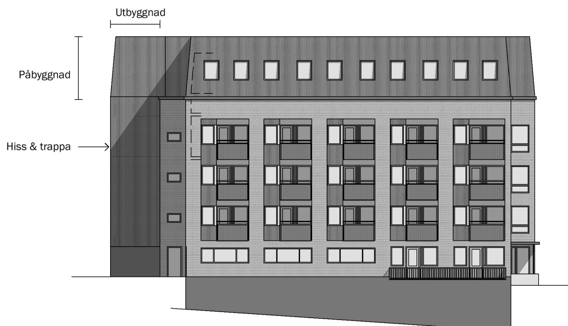
Nytt Fasad mot NV, Hus D Skala 1:250 (A3)
