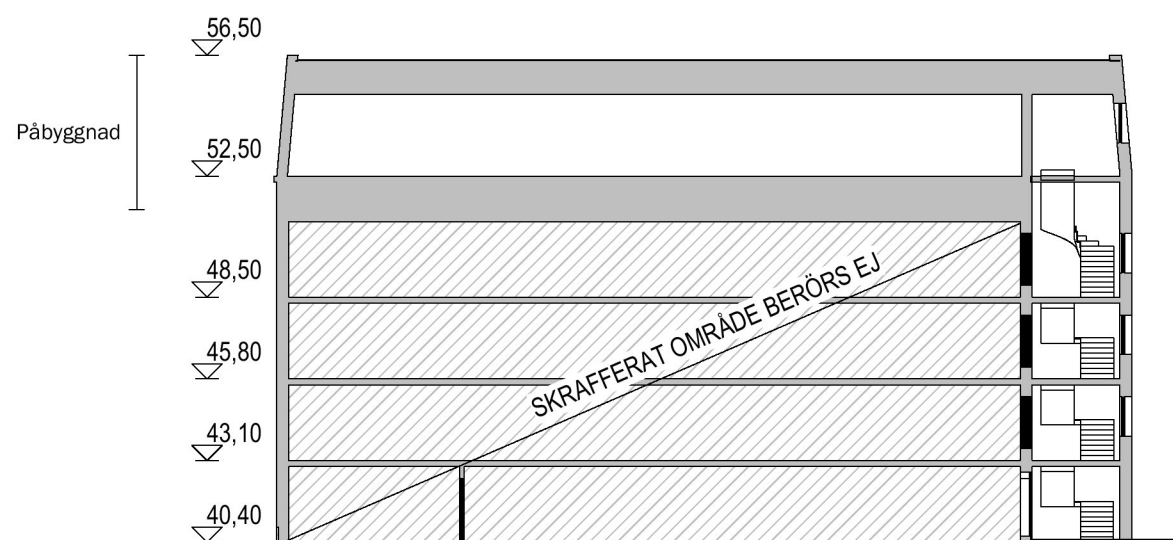
Nytt Sektion 5-5, Hus D Skala 1:250 (A3)
