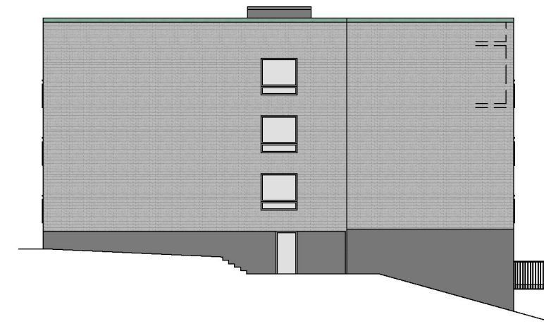
Befintligt Fasad mot NÖ, Hus D Skala 1:250 (A3)
