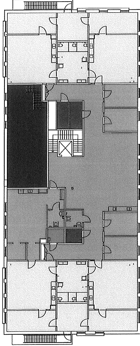
PLAN 200 Rutningen visar Sisabs typförskola "Framtidens förskola". Fönsterplacering och exakt placering av utrymningsstroppor anpassas till platsen.
