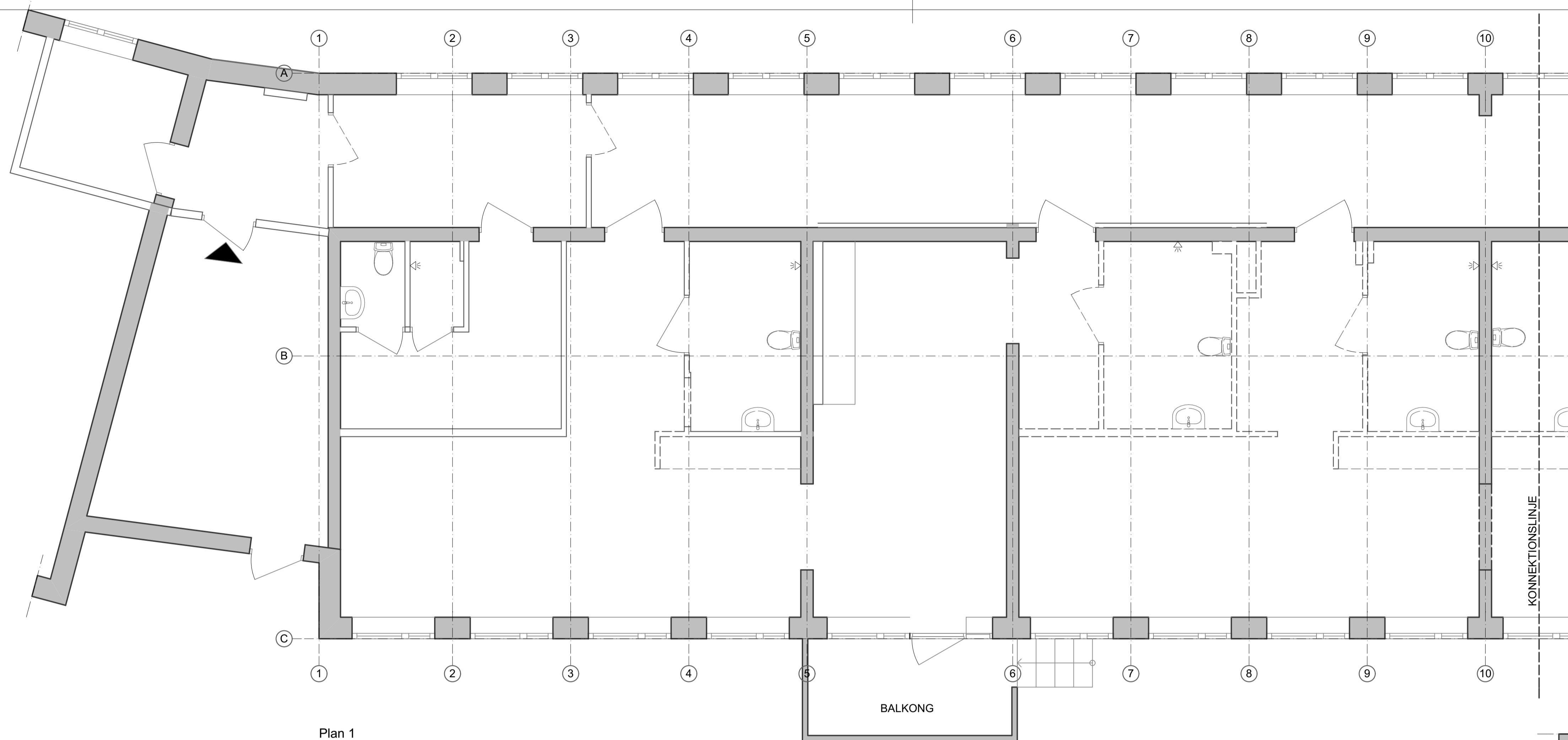
Plan 1 1:50
