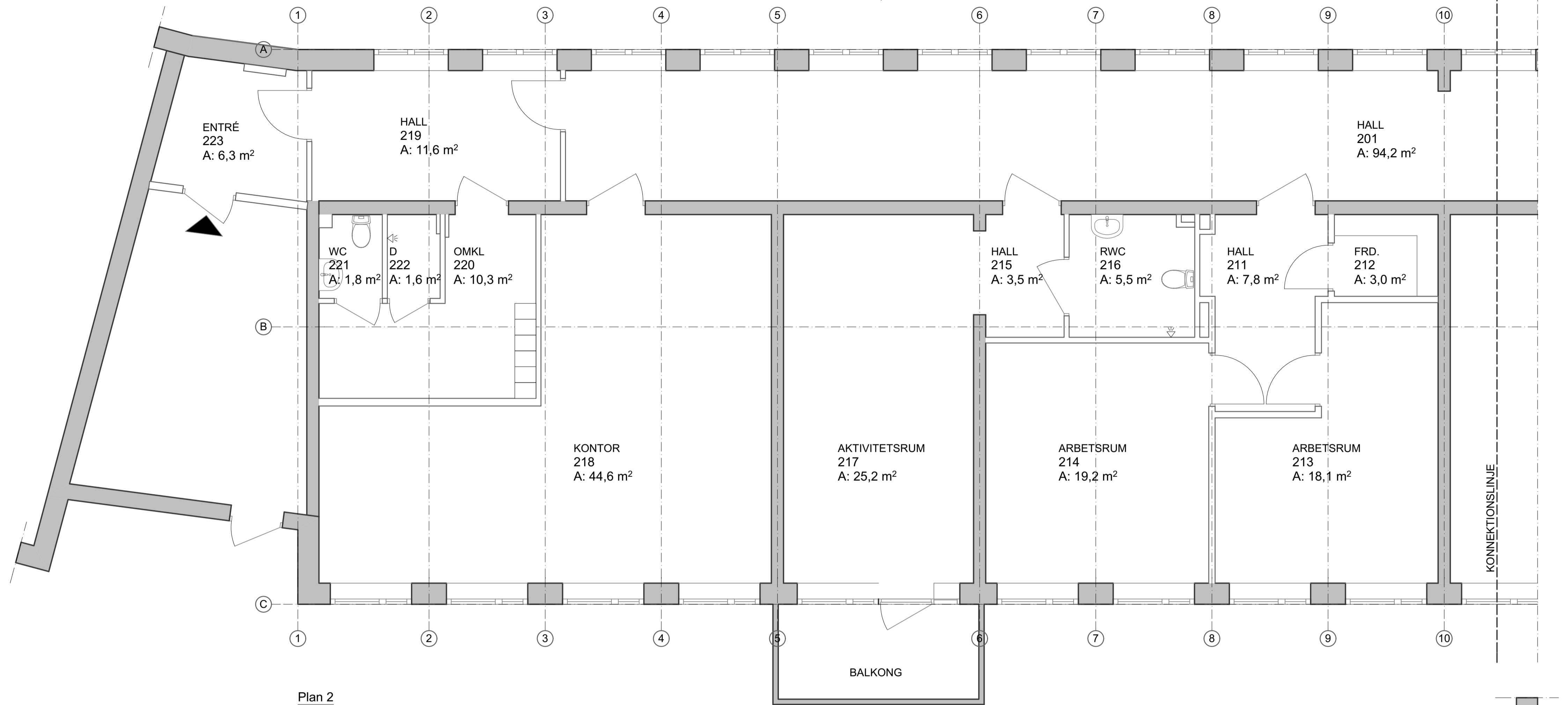
Plan 2 1:50
