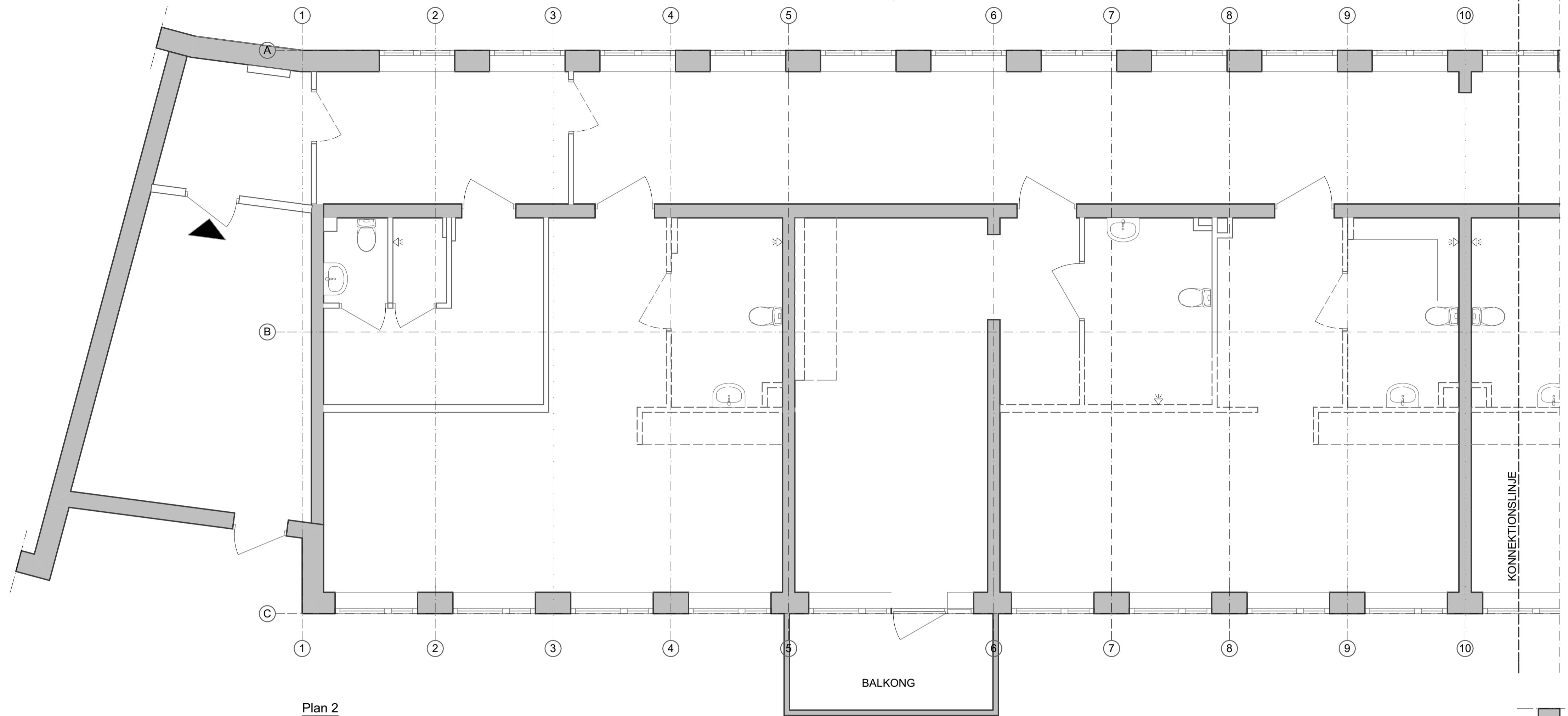
Plan 2 1:50
