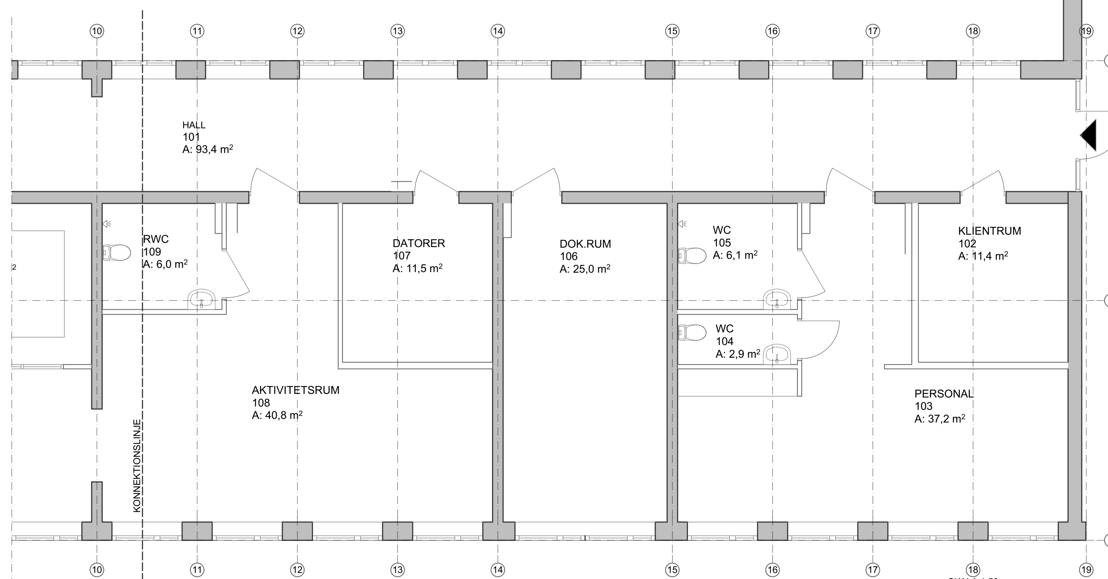
Plan 1 1:50
