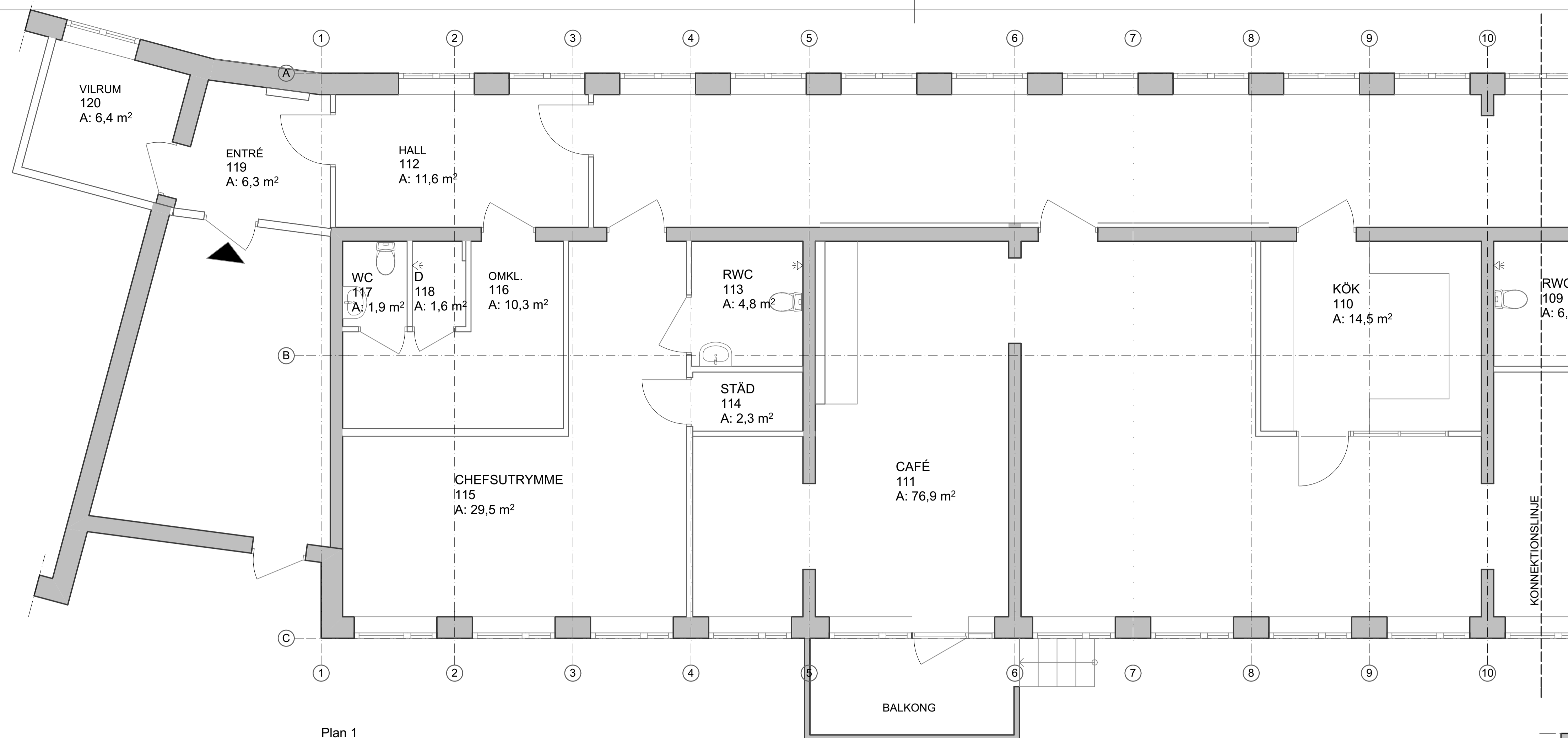
Plan 1 1:50
