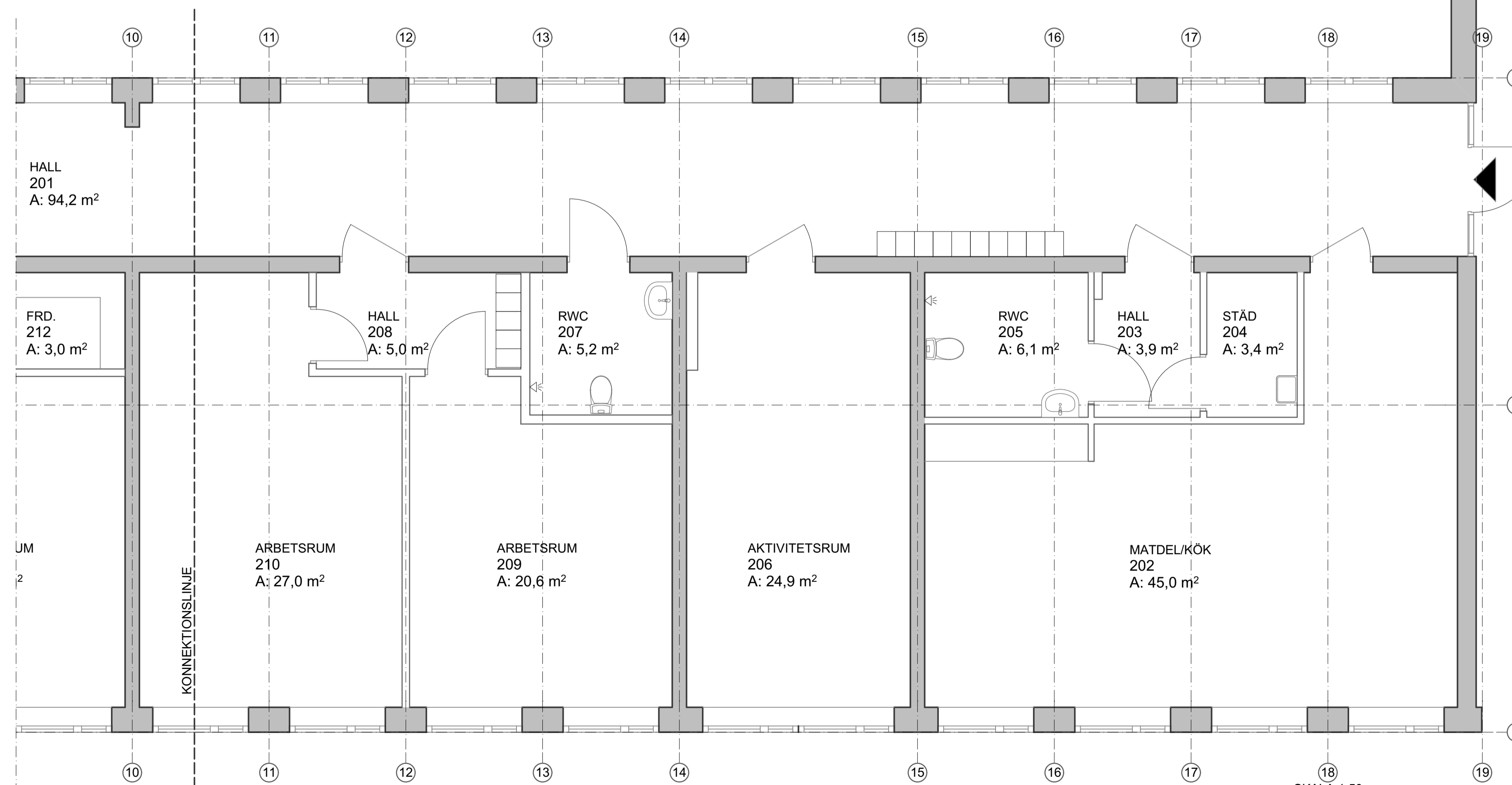
Plan 2 1:50
