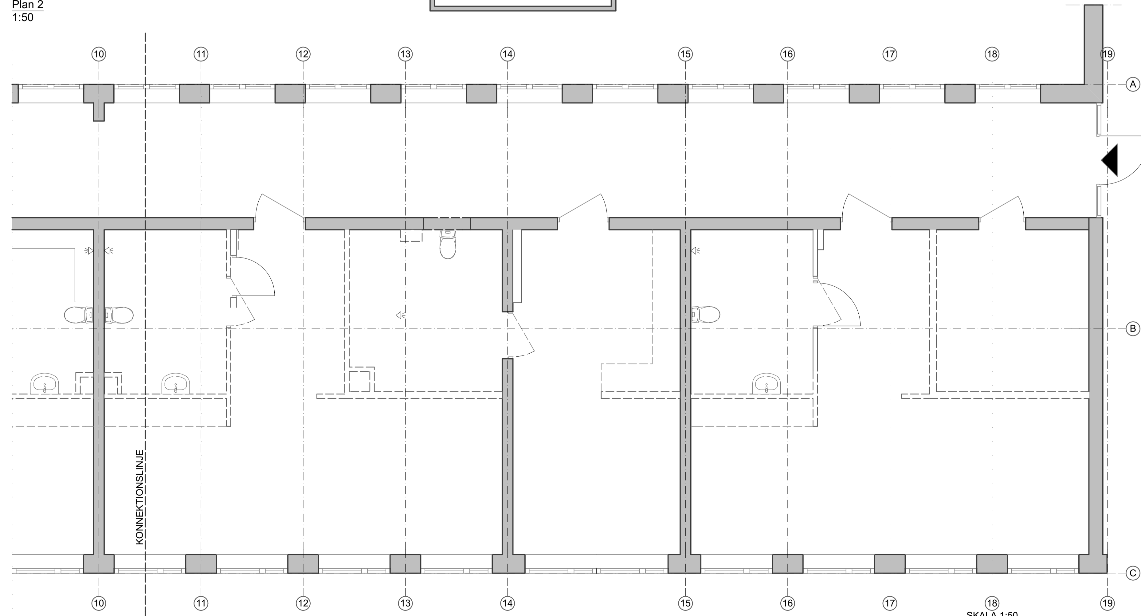
Plan 2 1:50
