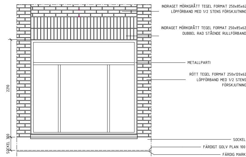
TV-2 TEGELDETALJ INDRAGET PARTI
