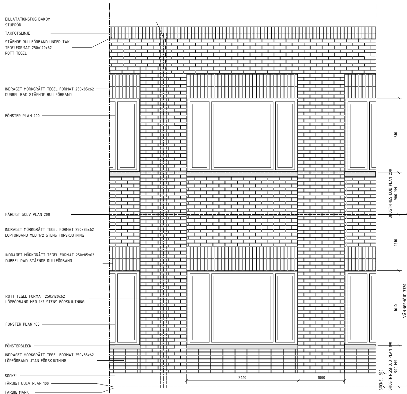
TV-1 TEGELDETALJ INDRAGNA FÖNSTER
