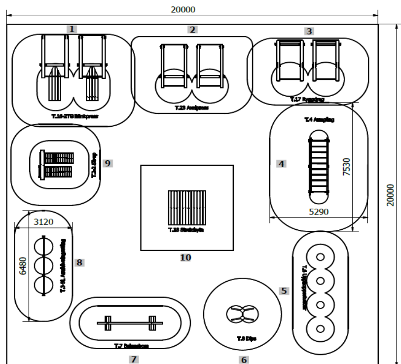
Bild 3. Planskiss utformning utegym anpassad efter platsen med yttermått 20 x 20 meter.
