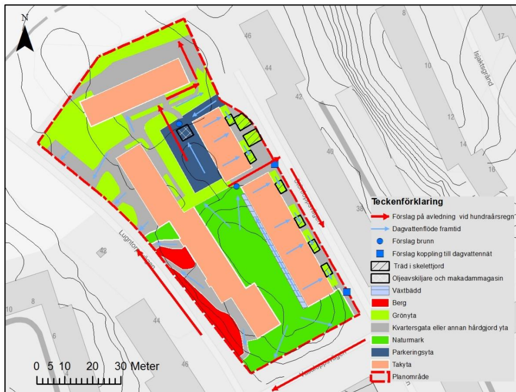
Figur 7-3. Förslag på avledning av dagvatten vid intensivt regn, såsom 100-årsregn (röda pilar)
