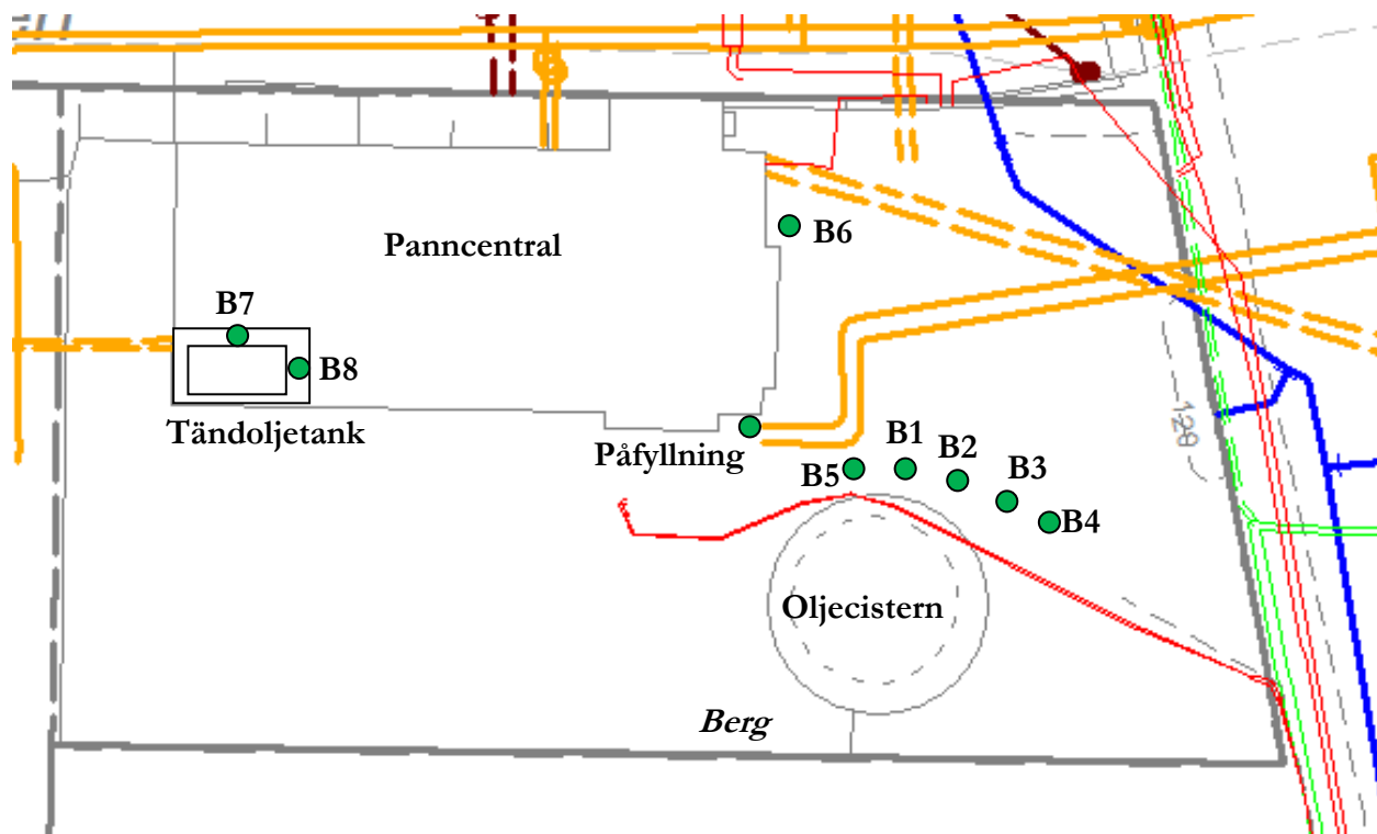
Figur 1. Provtagningsplan B1-B8.
