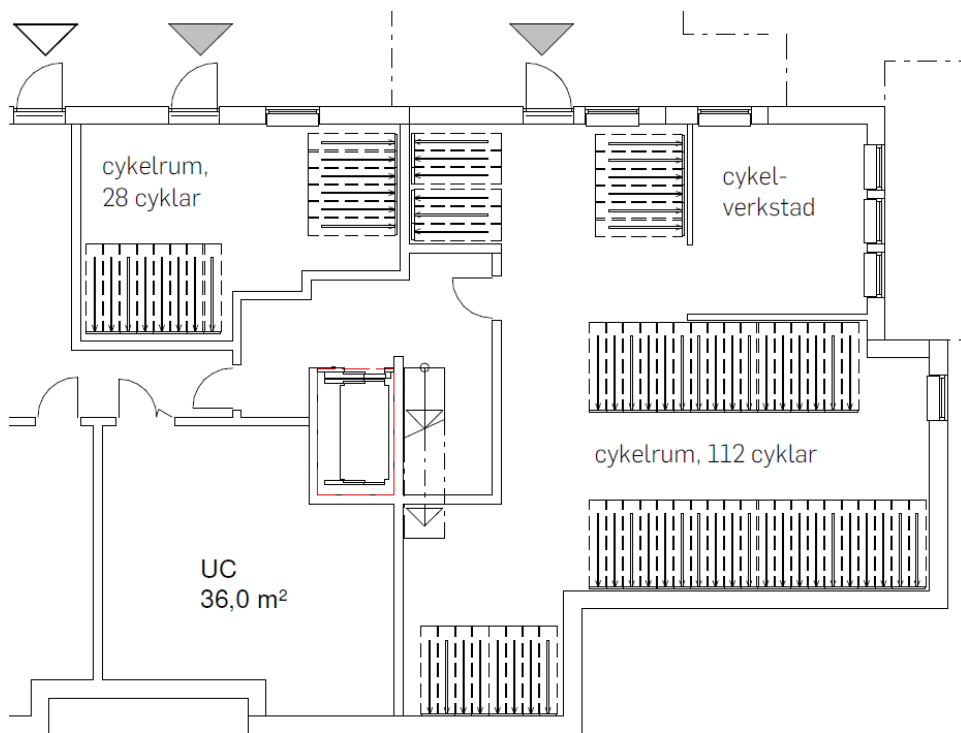
Figur 2-1 Kv. Norr: Ritning över källarplan med cykelrum och cykelverkstad. Källa: Lindberg Stenberg Arkitekter.
