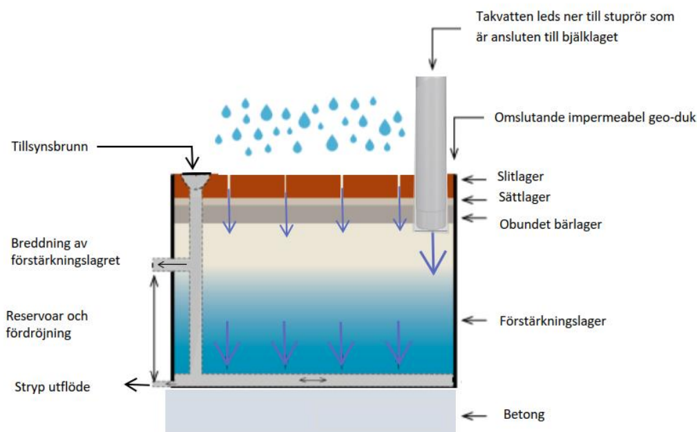
Figur 14. Principskiss (Inspiration från Svensk markbetong, 2019).
