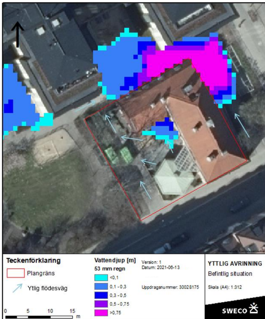
Figur 10. Lågpunktskartering inom planområdet med verktyget SCALGO Live och den ytliga flödesvägen vid skyfall.
