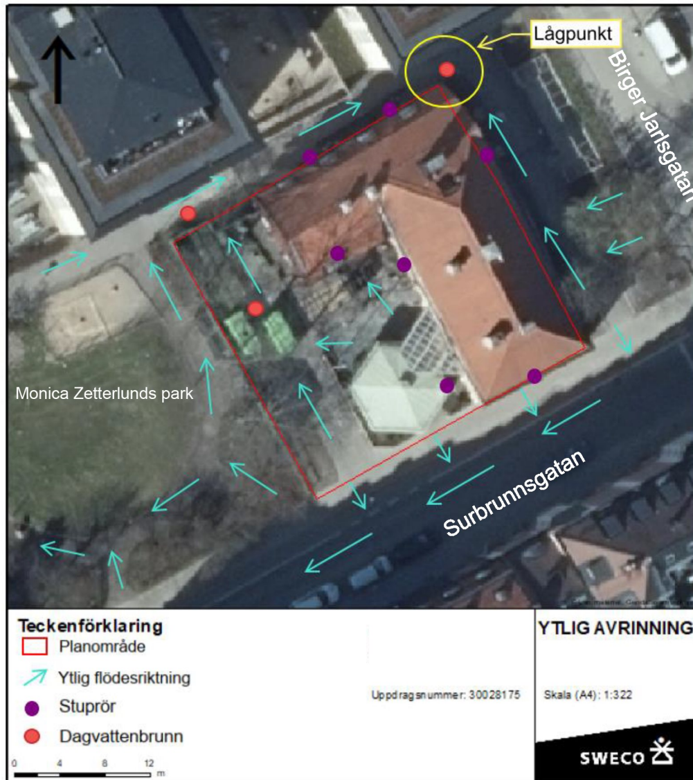
Figur 6. Ytavrinning inom planområdet, stuprören för avvattning av takvatten och de tre större dagvattenbrunnarna är utmarkerade i bilden. Dagvattenbrunnarna vid källaren tréer är ej utmarkerade.
