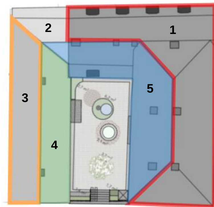
Figur 15. Uppdelning av takytor till respektive dagvattenåtgärd.
