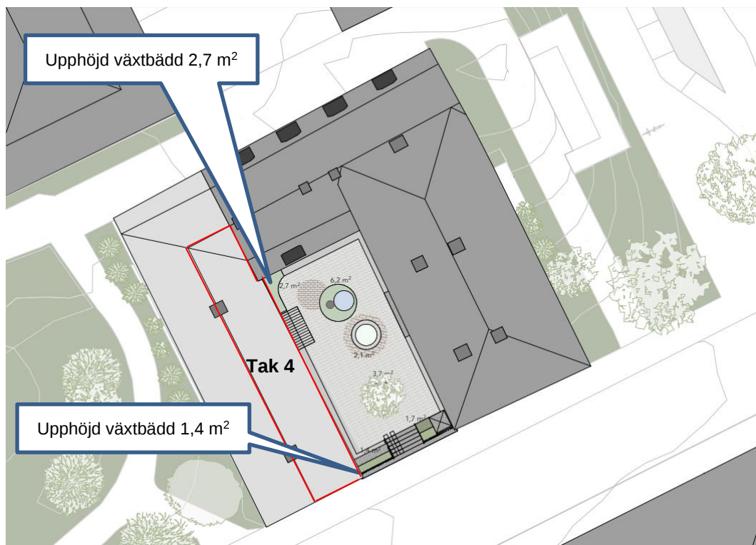
Figur 17. Placering av växtbäddar på innergården för avvattning av takyta 4. Föreslagen växtbäddsutbredning är totalt 4,1 m 2 .
