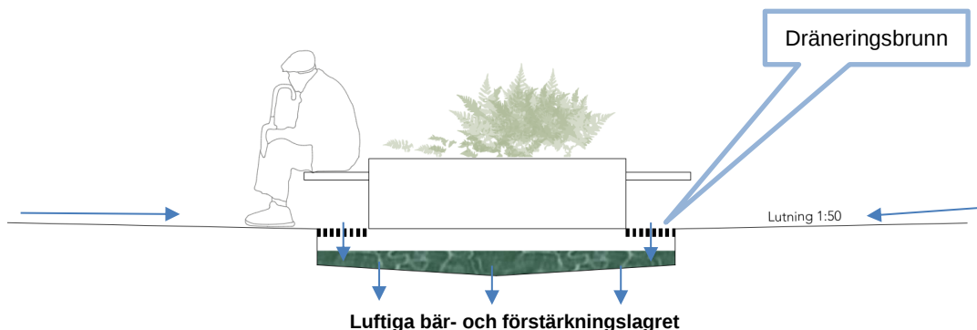
Figur 13. Dagvattnet som uppkommer på innergården avleds ytligt till dräneringsbrunnar som leder ner vattnet till en nedsänkt yta på innergården. Från den nedsänkta ytan avleds vattnet ner till luftiga bär- och förstärkningslager i bjälklaget. Vattnet som uppkommer på innergården ska även kunna infiltrera ner via fogarna på markplattorna till luftiga bär- och förstärkningslager i bjälklaget.
