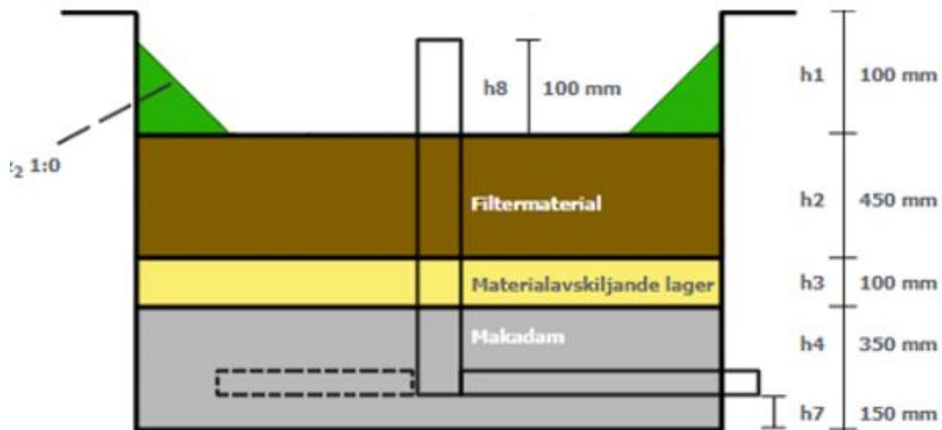
Figur 16. Principskiss på en växtbädd.
