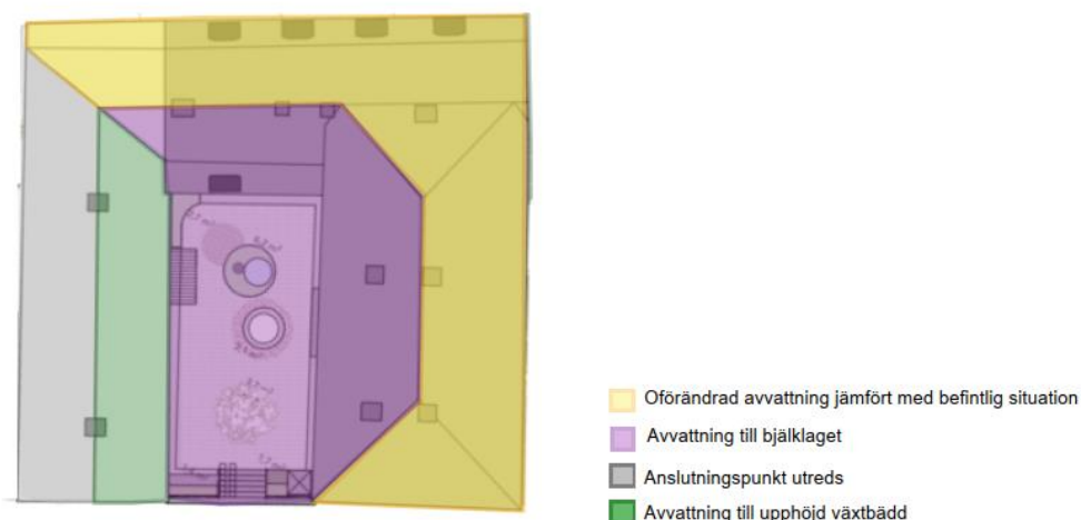
Figur 12. Konceptuella bild av åtgärdsförslagen och vilka ytor som avvattnas till vilken dagvattenlösning.
