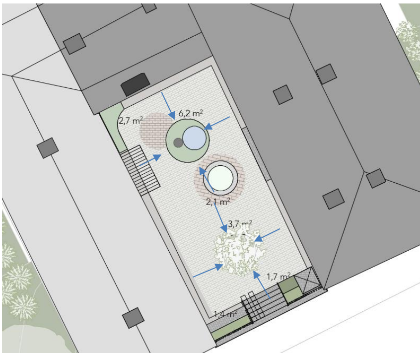
Figur 19. Konceptuell skiss över ytavrinningen till de nedsänkta ytorna som fungerar som förröjningsmagasin.
