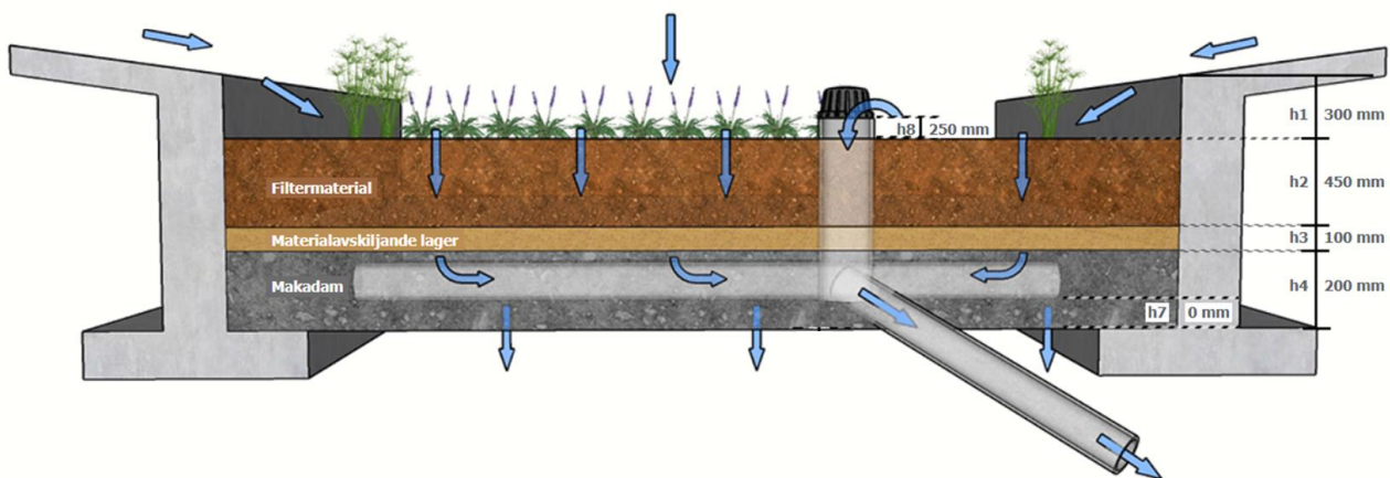
Figur 13. Principskiss på en växtbädd med underbyggnad och ytlig fördröjningsvolym. Växtbädden kan om förutsättningarna tillåtas vara otät (tillåta infiltration till mark).
