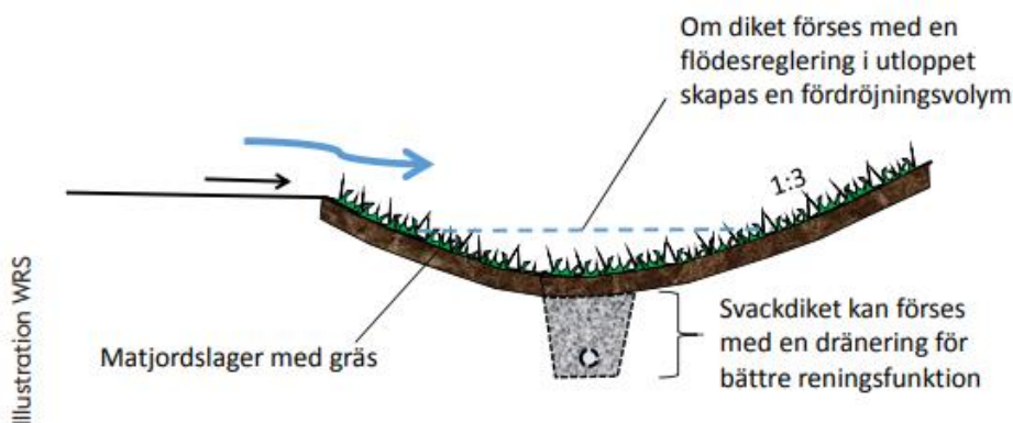
Figur 14. En principskiss för ett svackdike (Stockholm Vatten och Avfall - SVOA).
