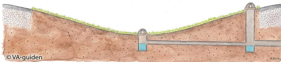
Figur 16. Skiss av en torr damm för dagvattenhantering (VA-guiden).
