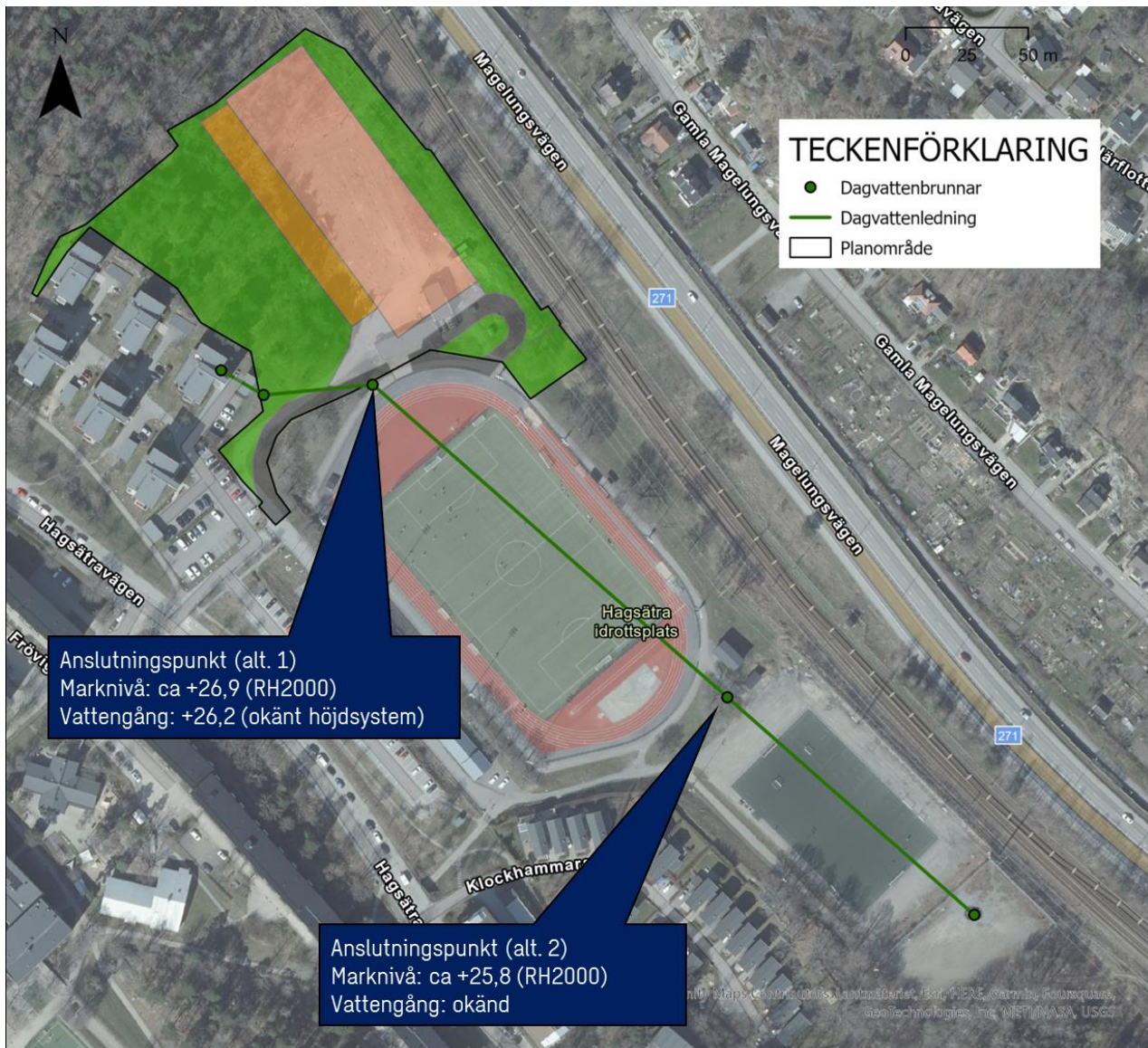
Figur 20. Befintliga dagvattenledningar och brunnar i och i närheten av planområdet. Marknivåer presenteras i RH2000, vattengången i dagvattenbrunnen (alt.1) är mätt i okänt höjdsystem. Figuren visar två möjliga anslutningspunkter för dagvatten.
