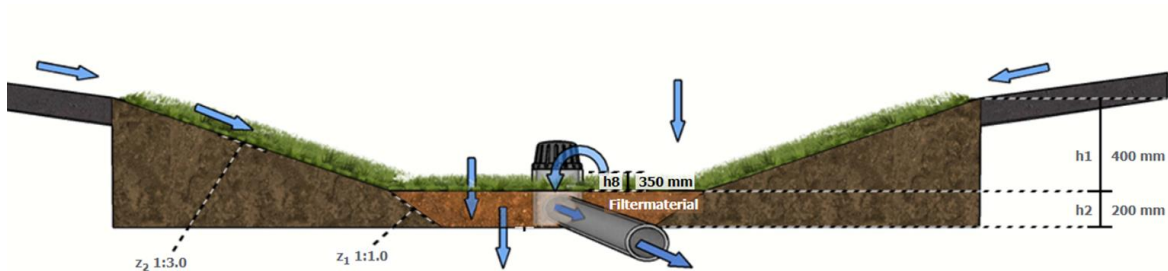
Figur 15. Dimensioner för det föreslagna svackdiket.
