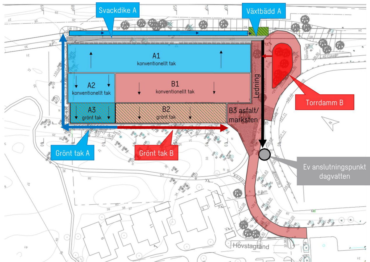
Figur 19. Översiktlig systemlösning för dagvattenhantering.
