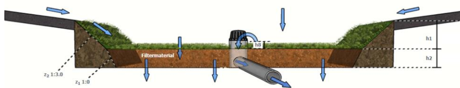
Figur 17. Dimensioneringskiss torrdamm.
