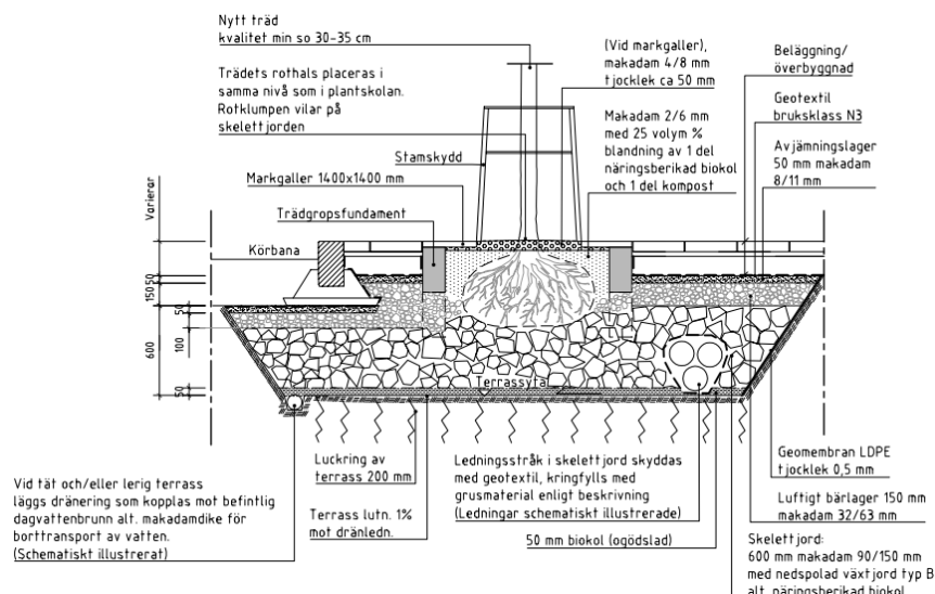
Figur 16. Principskiss skelettjord med träd i hårdgjord yta (Stockholms stad, 2017).
