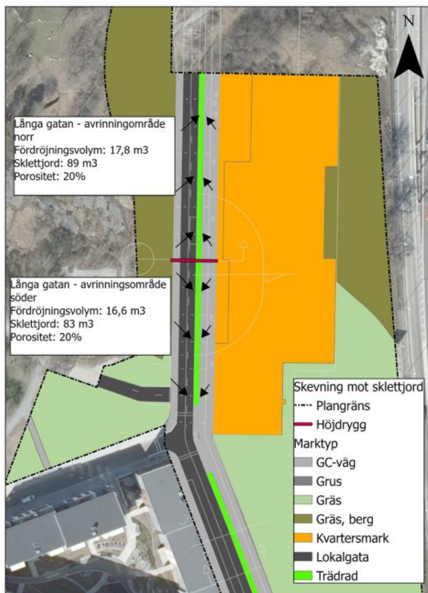
Figur 17. Föreslagen dagvattenhantering och avvattningsplan.
