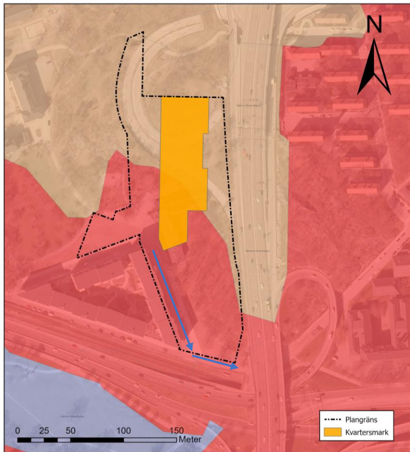
Figur 10. Befintliga tekniska avrinningsområden (enligt SVOA:s öppna geodata) och översiktliga rinnvägar längs dagvattenledning är markerat i blått.
