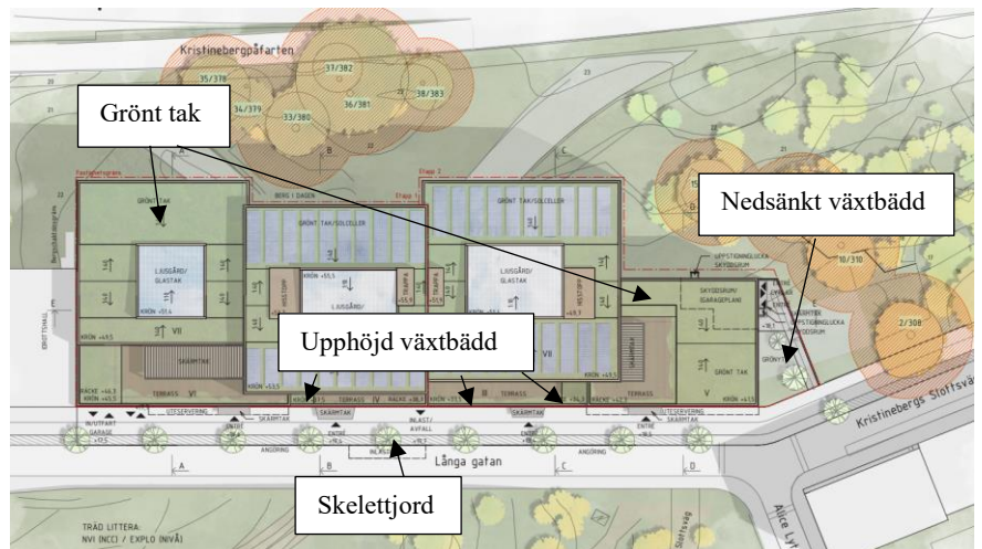
Figur 18. Illustration över föreslagna dagvattenanläggningar för allmän platsmark och kvartersmark. (White, 2023)
