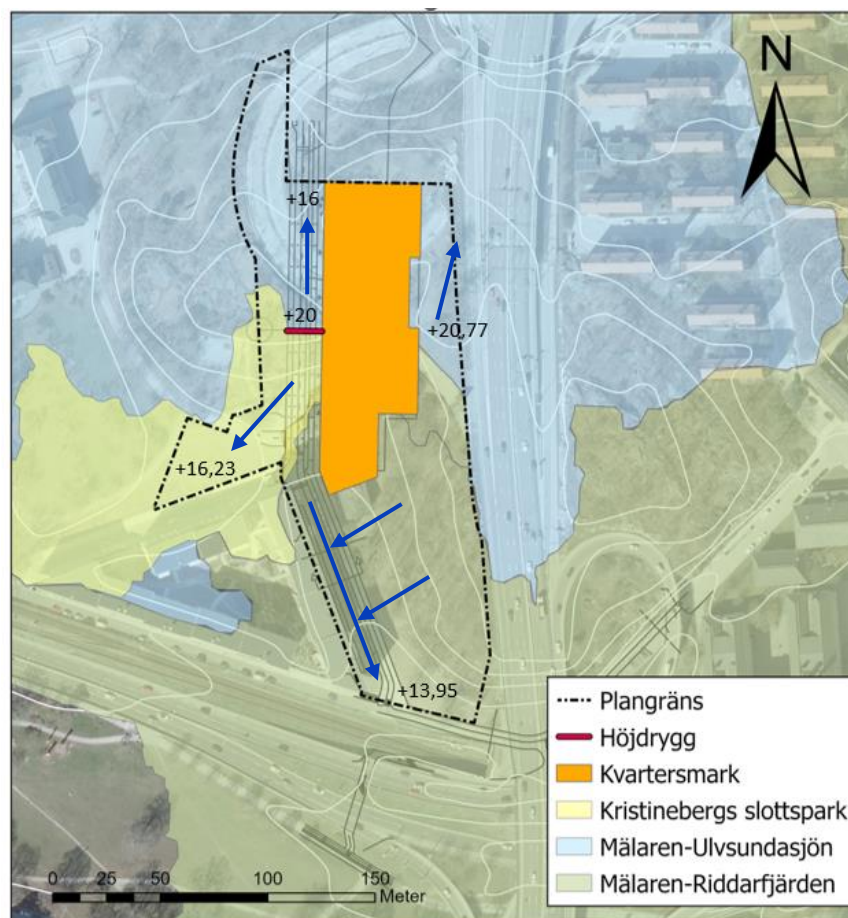
Figur 9. Ytliga avrinningsområden för planerat scenario (enligt SCALGO Live, 2023). Blå pilar visar på översiktliga rinnvägar inom utredningsområdet.
