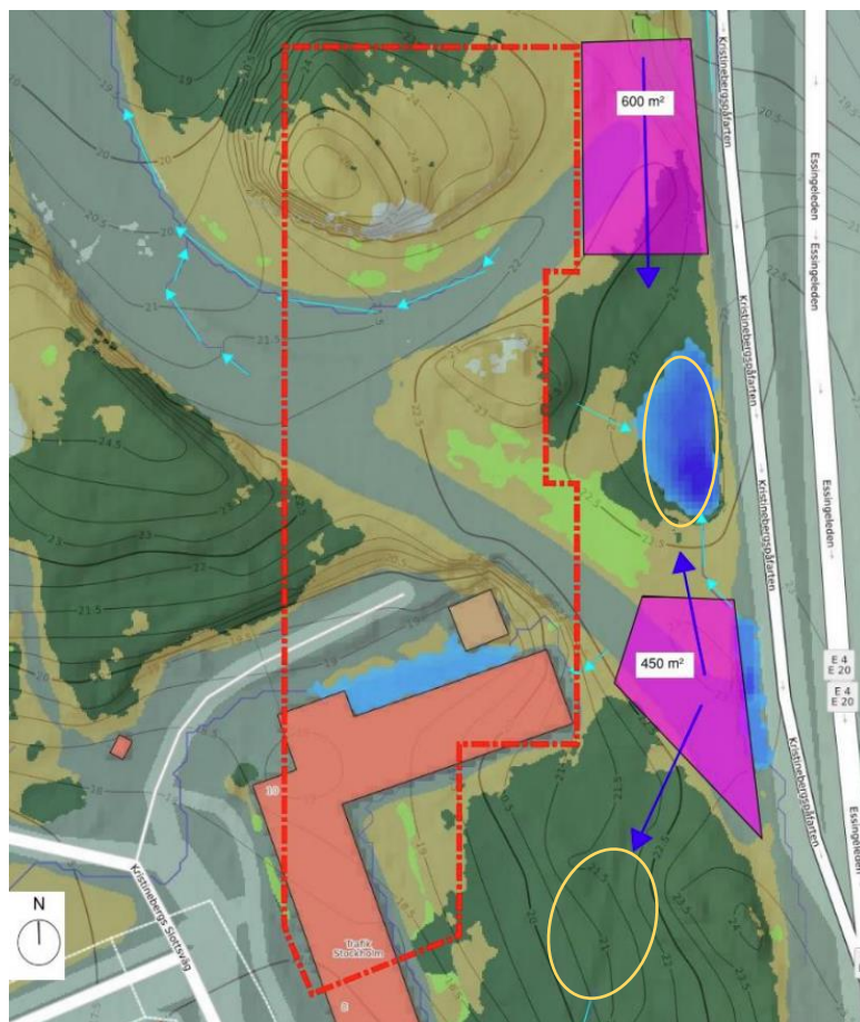
Figur 15. Topografisk karta från Scalgo LIVE. Rosa partier motsvarar ytor på allmän platsmark som ev. kan lutas mot ekar för att kompensera för det vatten som omhändertas inom fastigheten Kristineberg 1:10. Turkos flödespilar motsvarar flödesriktningen som enligt SCALGO sker naturligt utifrån befintliga markförhållanden. Ekarnas placering är inringat i gult. (Incoord, 2023)
