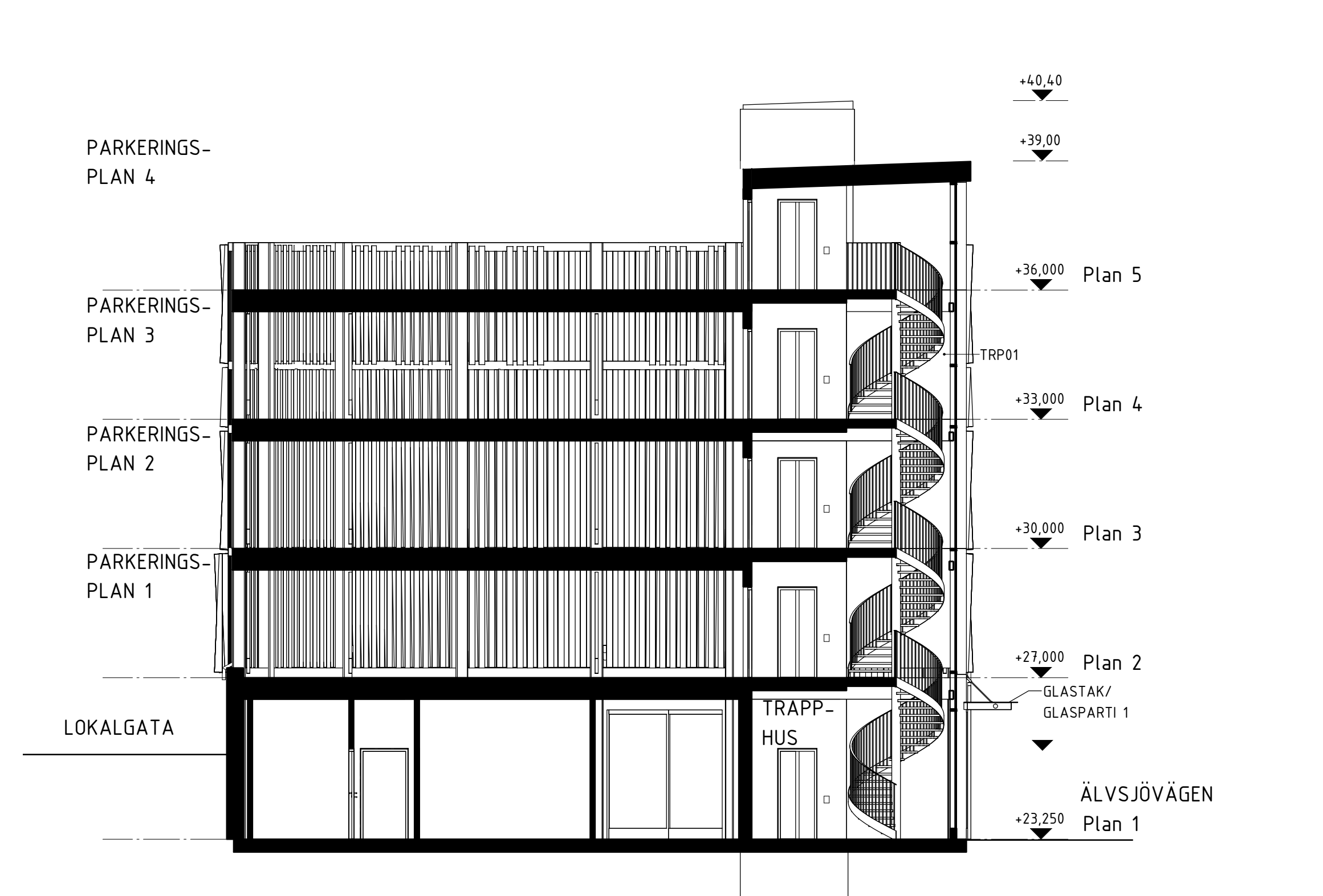
SEKTION C-C
