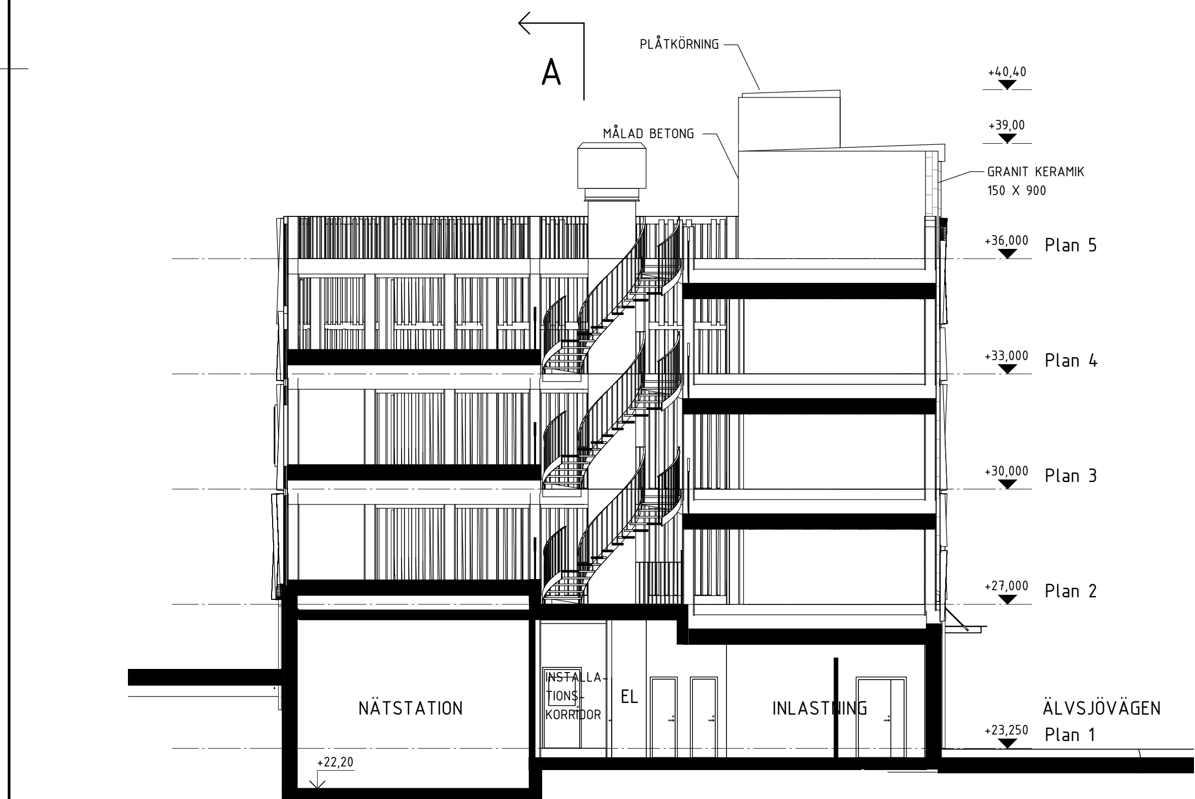
SEKTION A-A
