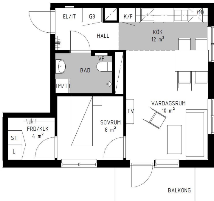
Bild 1. Planlösning 2 rok 44 kvm
