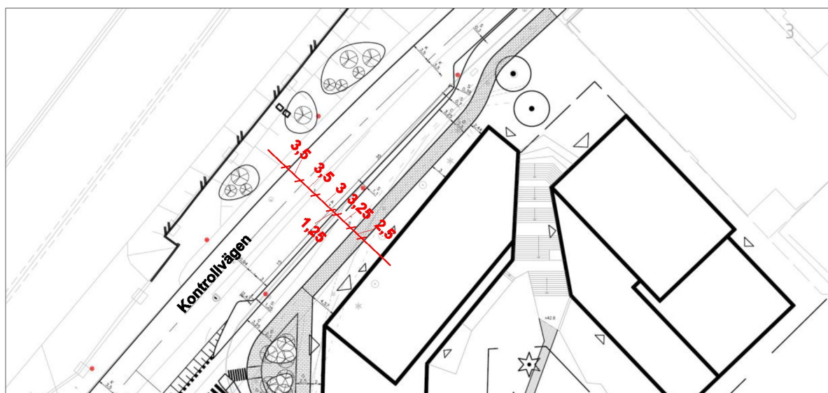
Figur 10 Kontrollvägen
